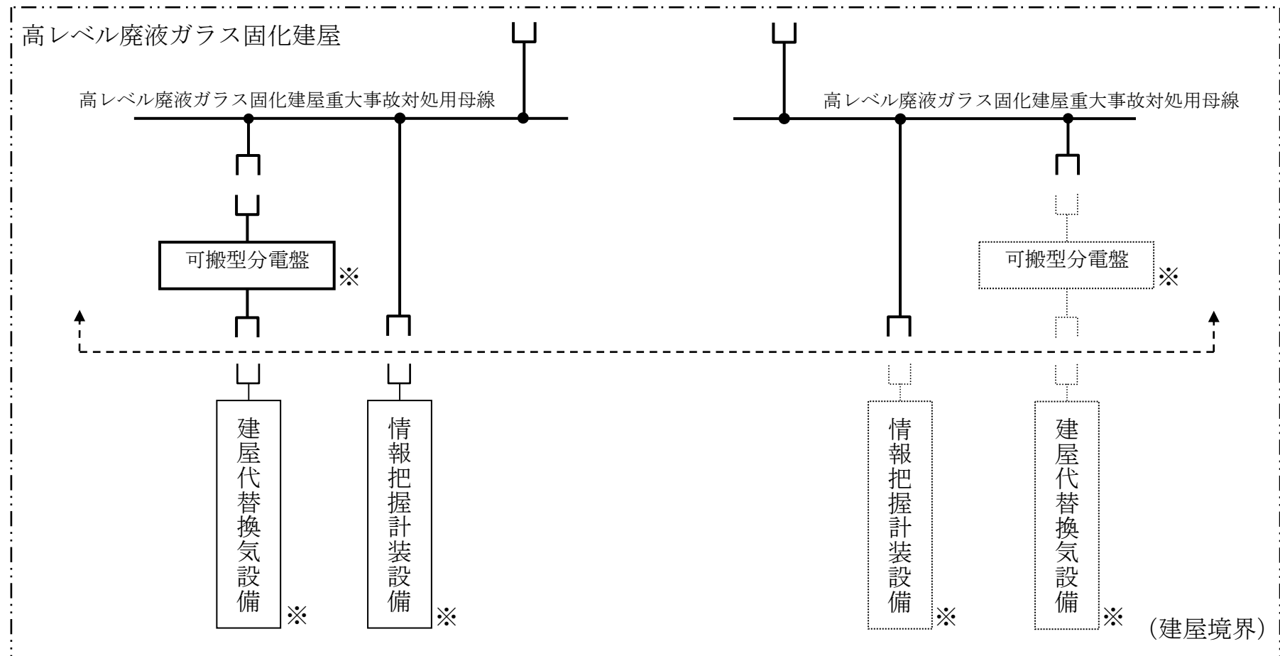
第 1.10-4 図 電源設備の単線結線図 (高レベル廃液ガラス固化建屋可搬型発電機～高レベル廃液ガラス固化建屋重大事故対処用母線) (6 / 8)
