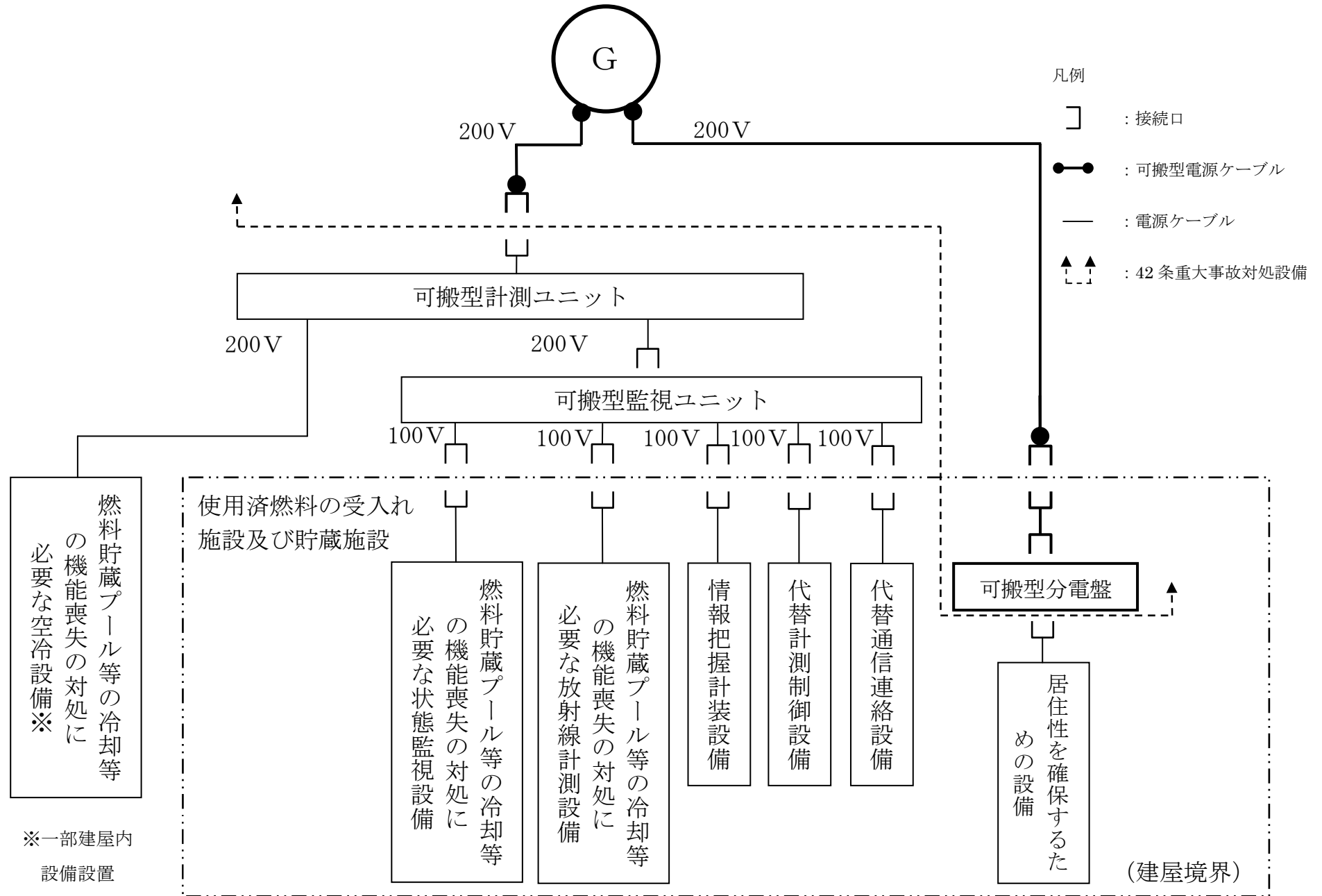
第 1.10-4 図 電源設備の単線結線図 (可搬型発電機～使用済燃料の受入れ施設及び貯蔵施設) (8 / 8)
