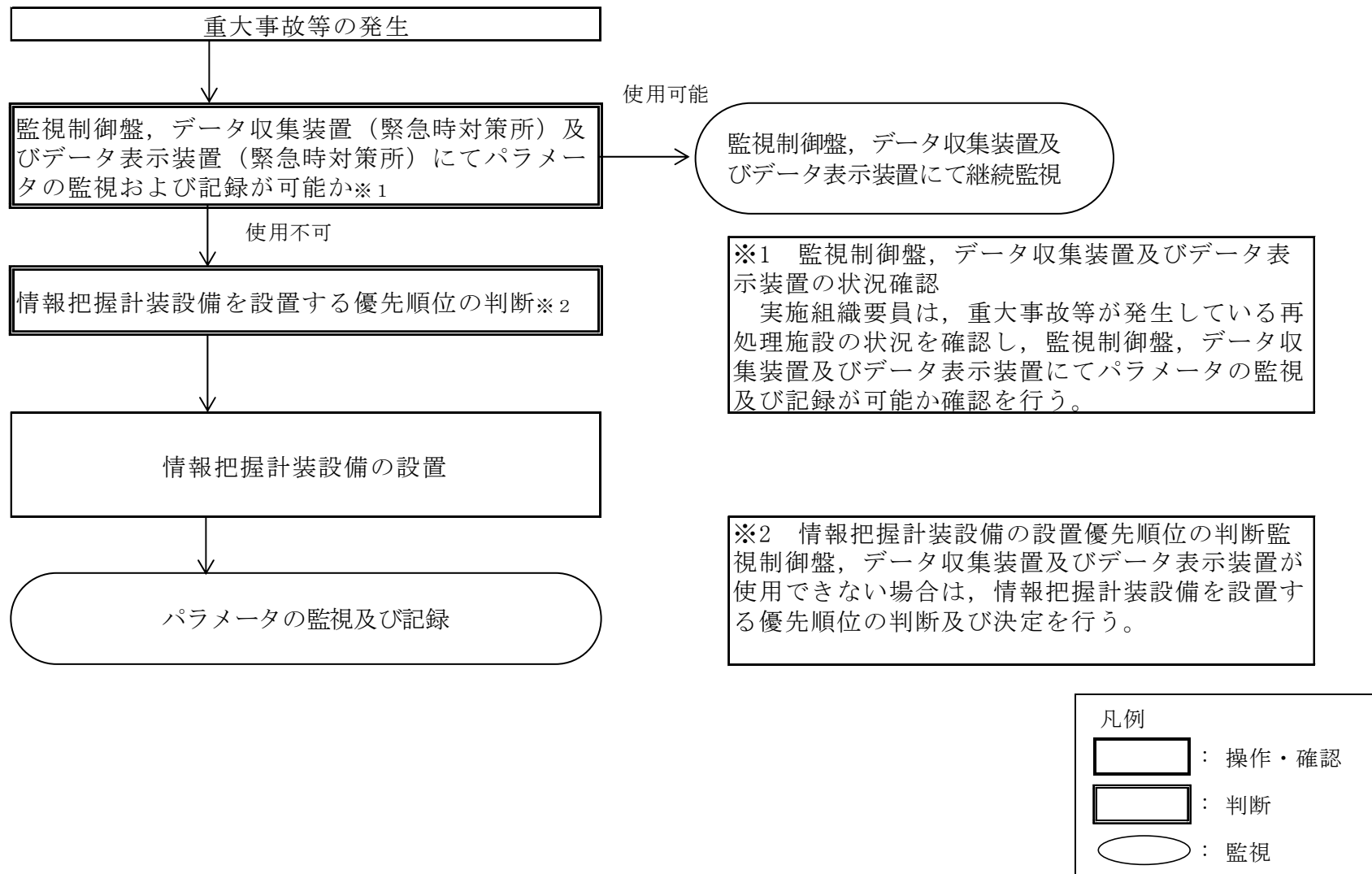
第 1.10-6 図 重大事故等時のパラメータを監視及び記録する手順
