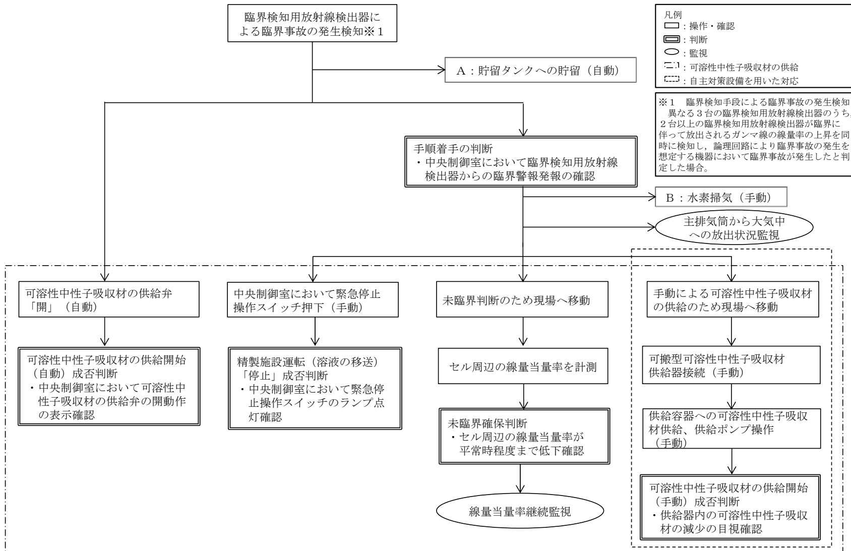
第7図 「精製建屋における臨界事故」の手順の概要 (1/2)
