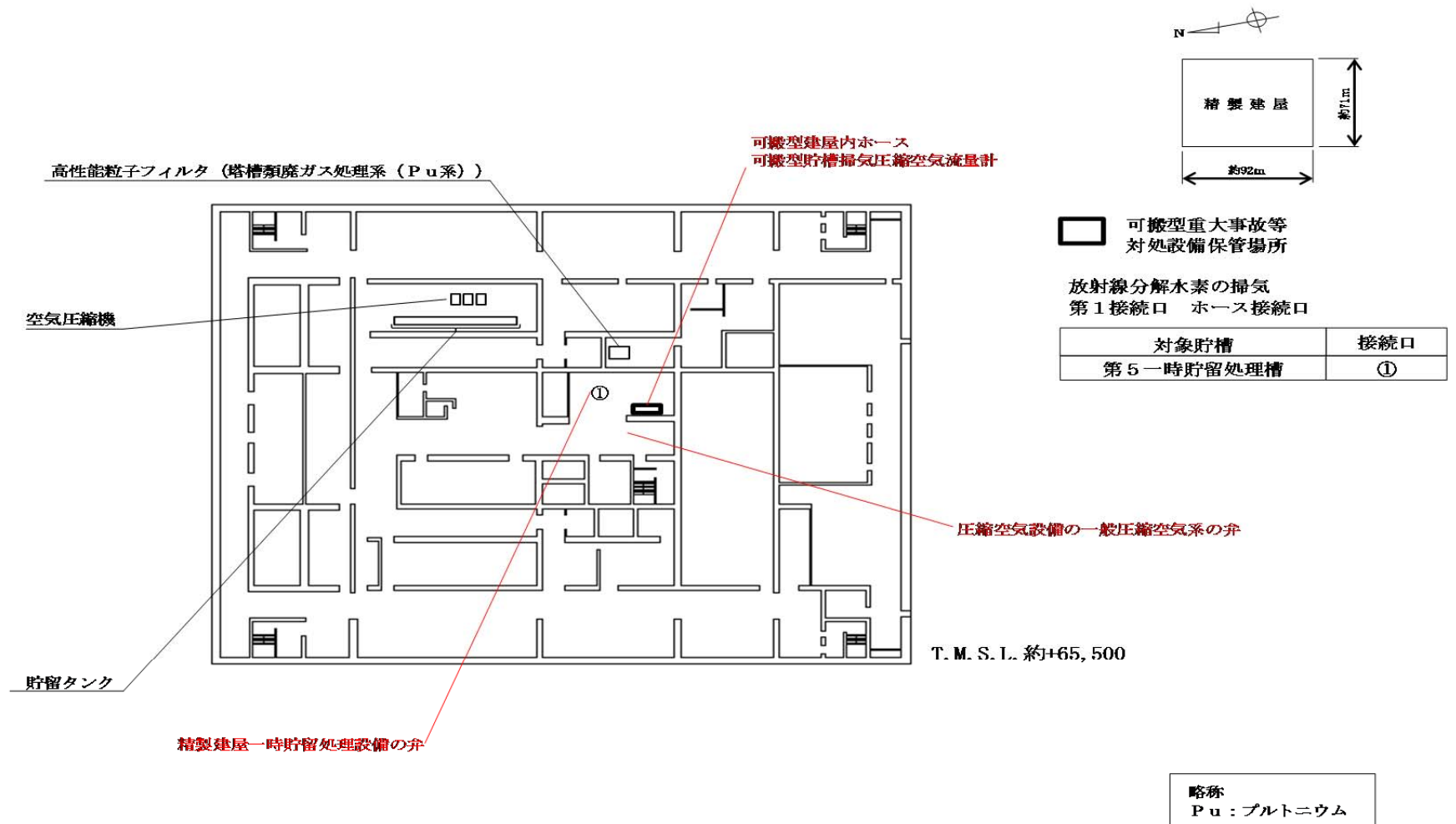
精製建屋 臨界事故の拡大防止のための措置の機器配置概要図 (地上4階) (放射線分解水素の掃気)
