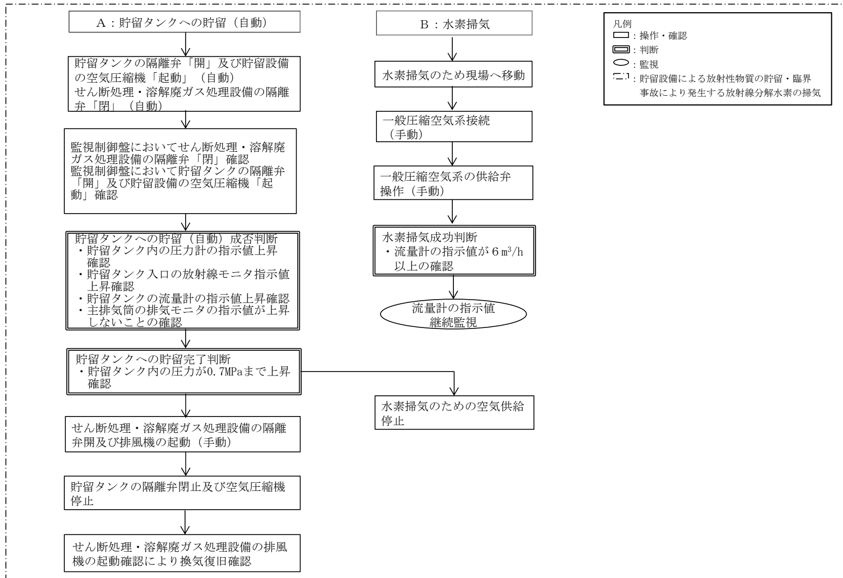
第1図 「前処理建屋における臨界事故」の手順の概要 (2/2)
