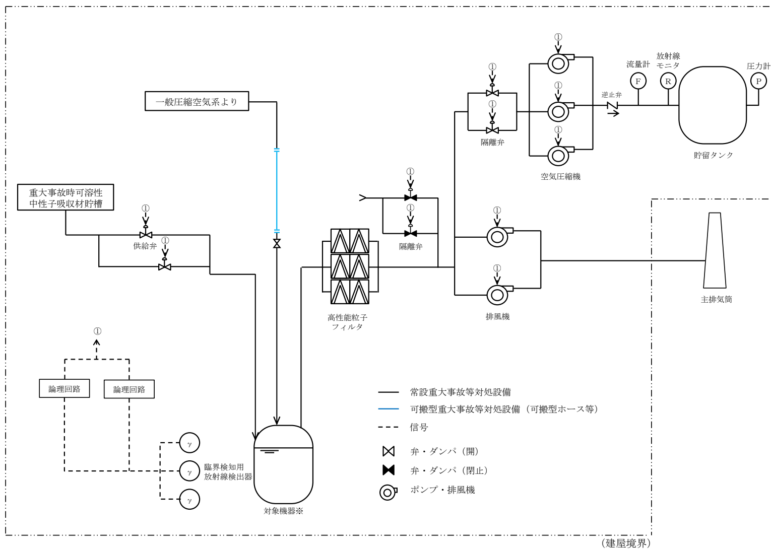
第 2.1-2 図 精製建屋 臨界事故の拡大防止のための措置の系統概要図 (1 / 2)
