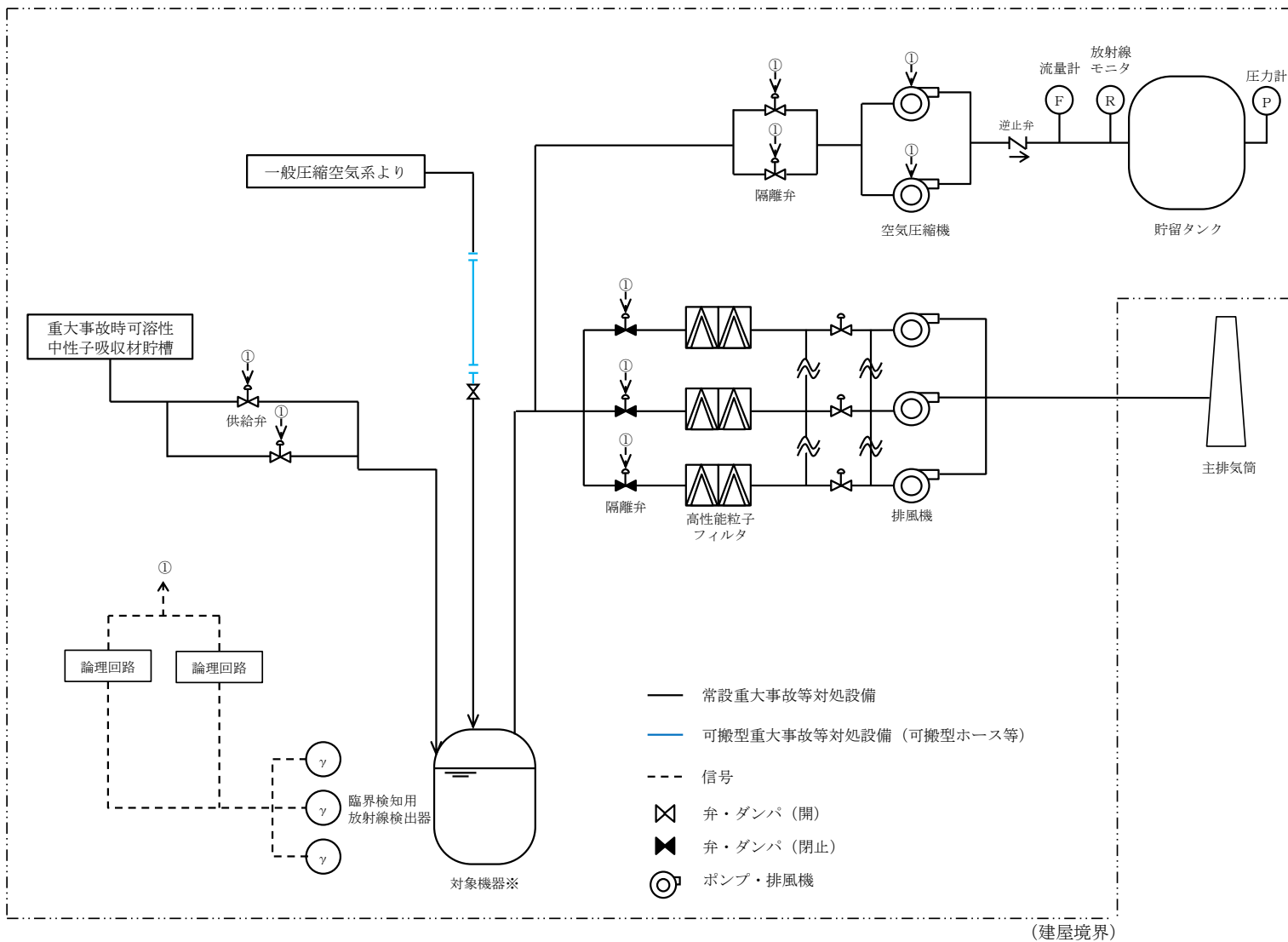
第 2.1-1 図 前処理建屋 臨界事故の拡大防止のための措置の系統概要図 (1 / 2)
