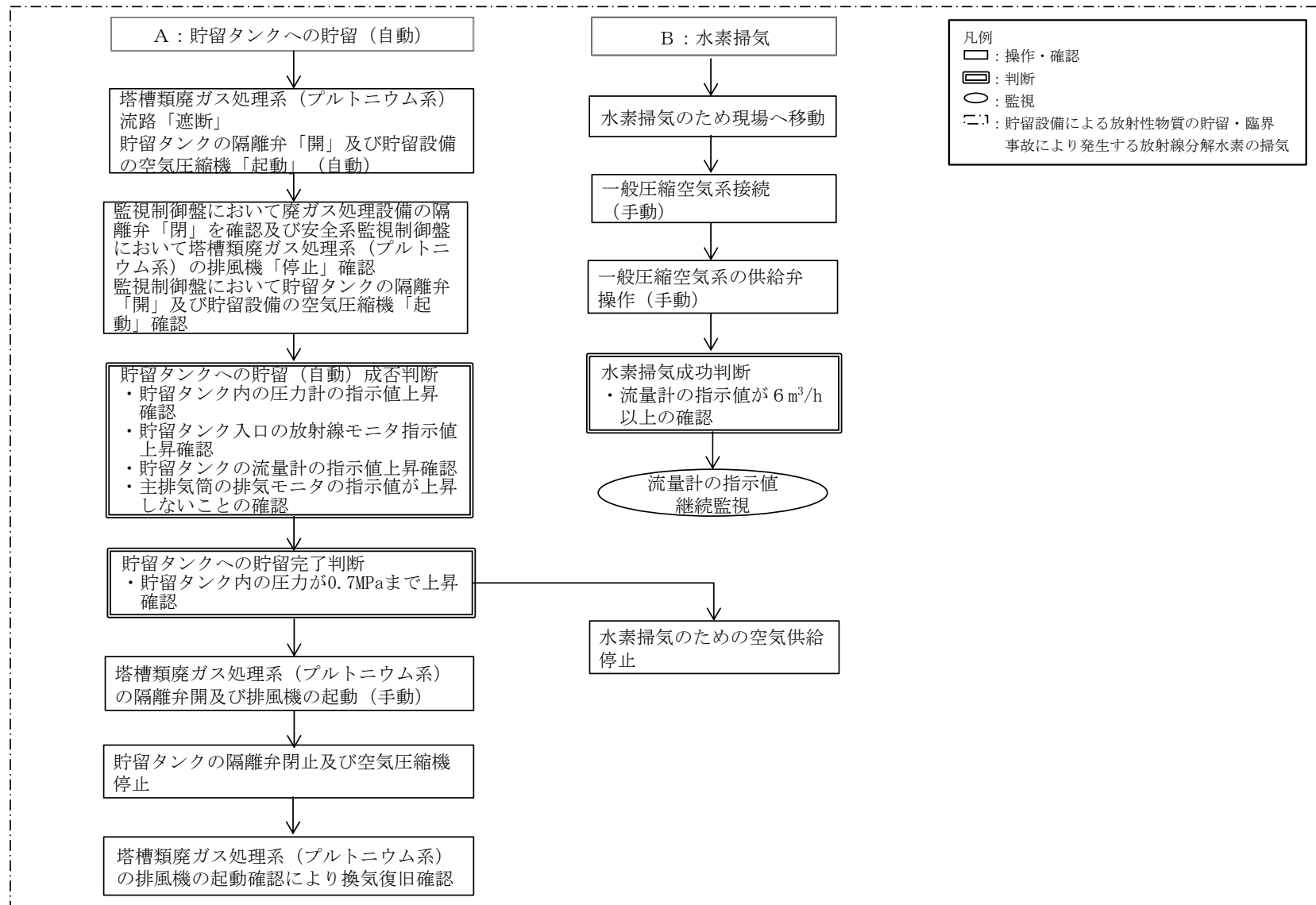
第7図 「精製建屋における臨界事故」の手順の概要 (2/2)
