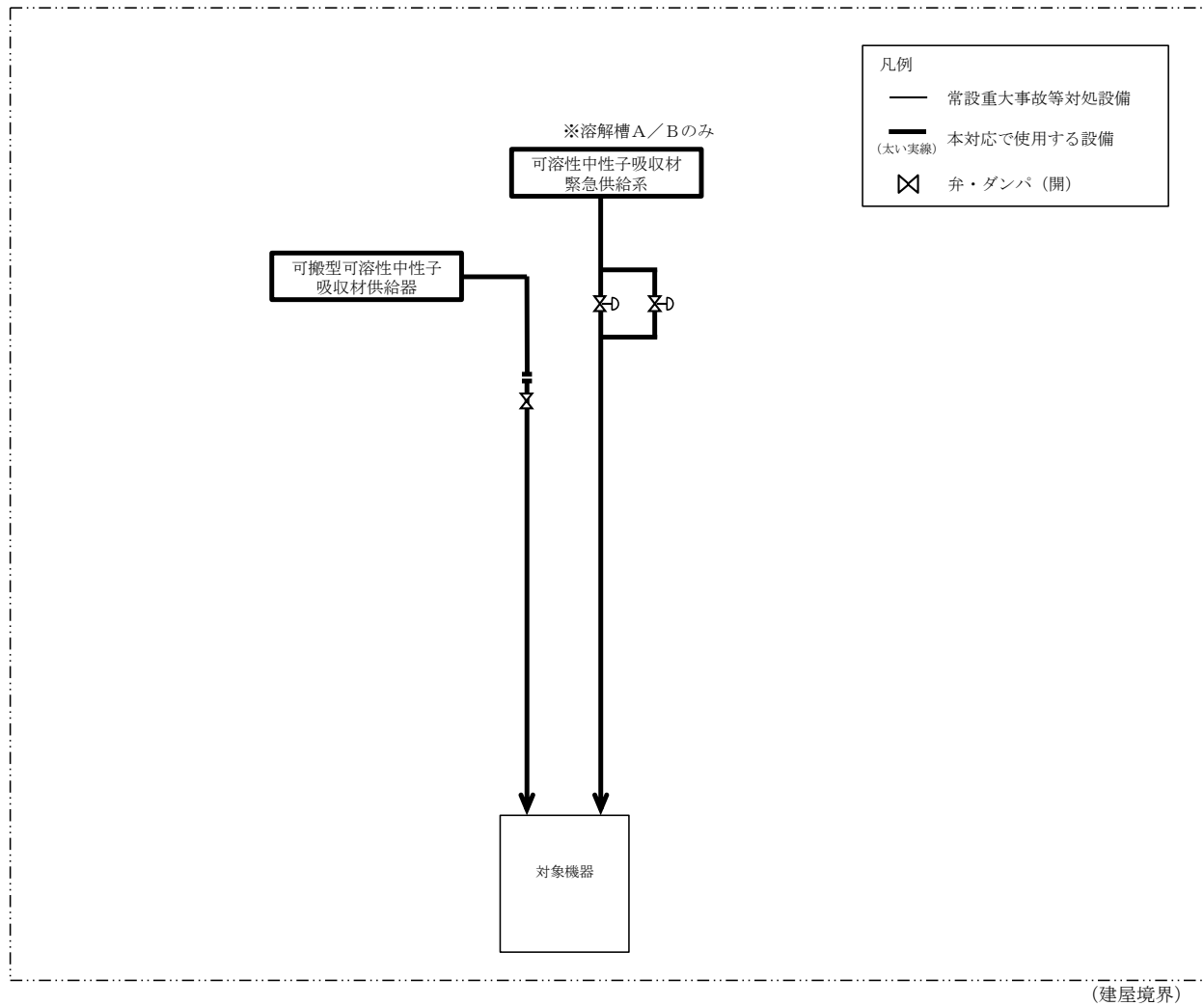
第2図 前処理建屋 臨界事故の拡大防止のための措置の系統概要図 (自主対策設備を用いた可溶性中性子吸収材の供給)
