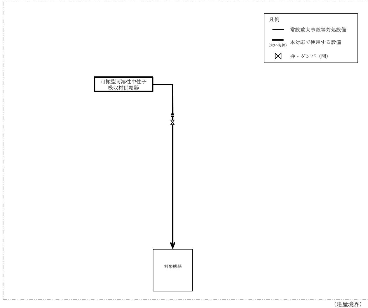
第8図 精製建屋 臨界事故の拡大防止のための措置の系統概要図 (自主対策設備を用いた可溶性中性子吸収材の供給)
