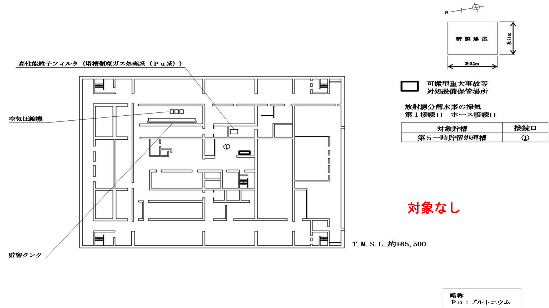
精製建屋 臨界事故の拡大防止のための措置の機器配置概要図 (地上4階) (貯留設備による放射性物質の貯留)
