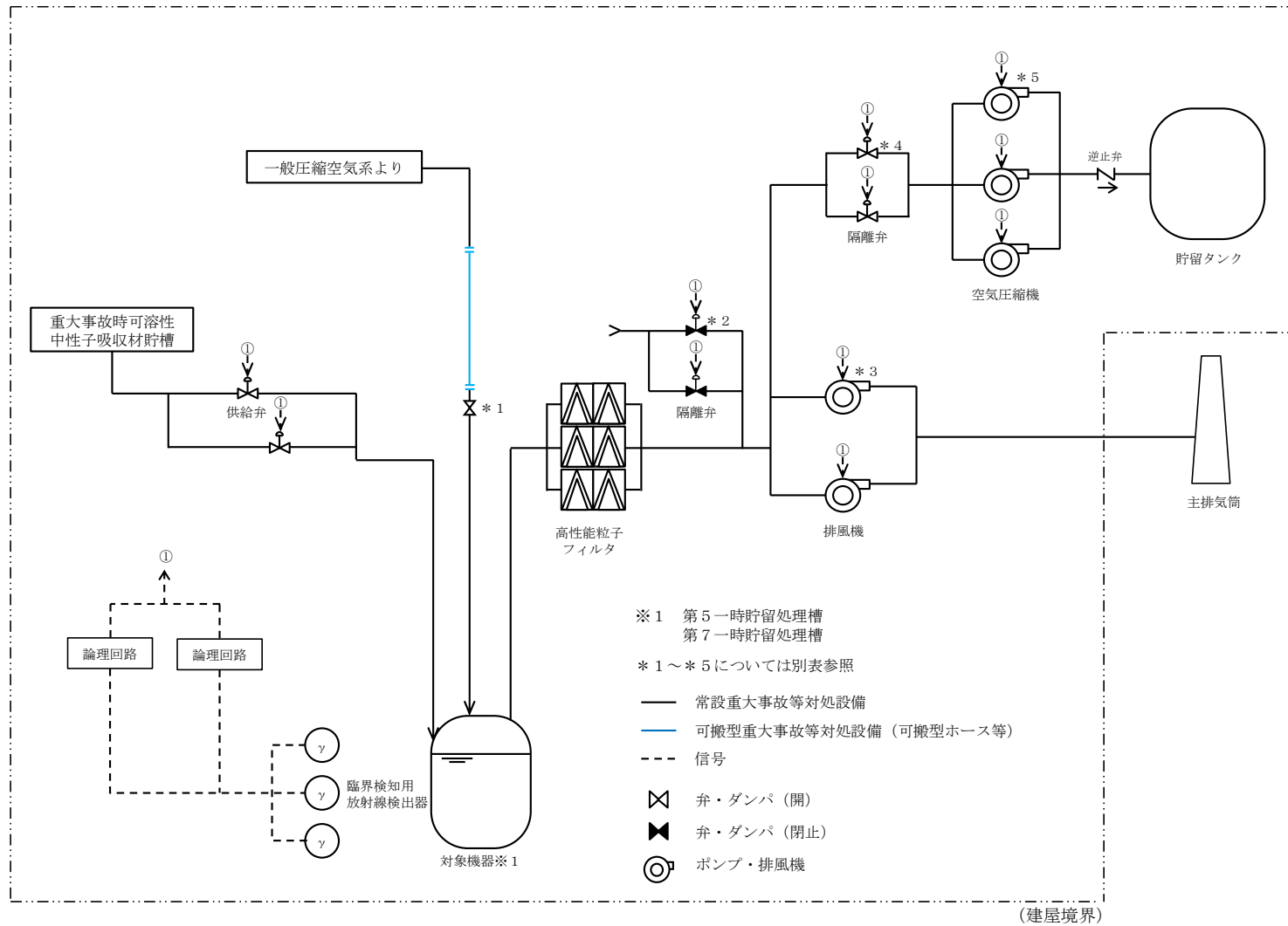
精製建屋における臨界事故の拡大を防止するための設備の系統概要図
