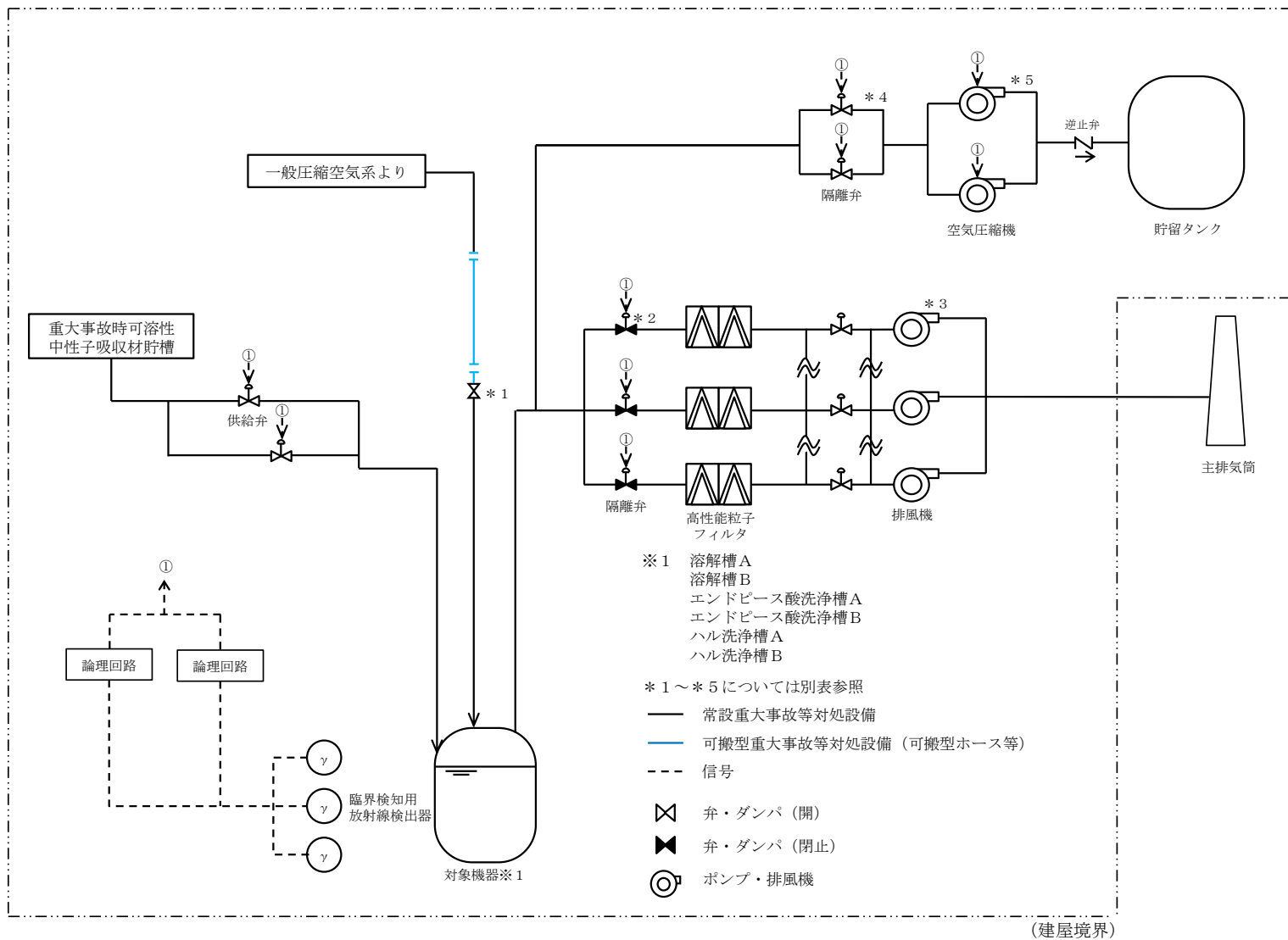
前処理建屋における臨界事故の拡大を防止するための設備の系統概要図
