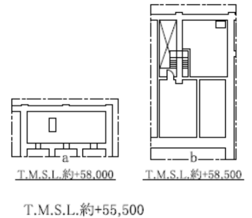
第 2.1-3 図 前処理建屋 臨界事故の拡大防止のための措置の接続口位置図 ( 1 / 2 )
