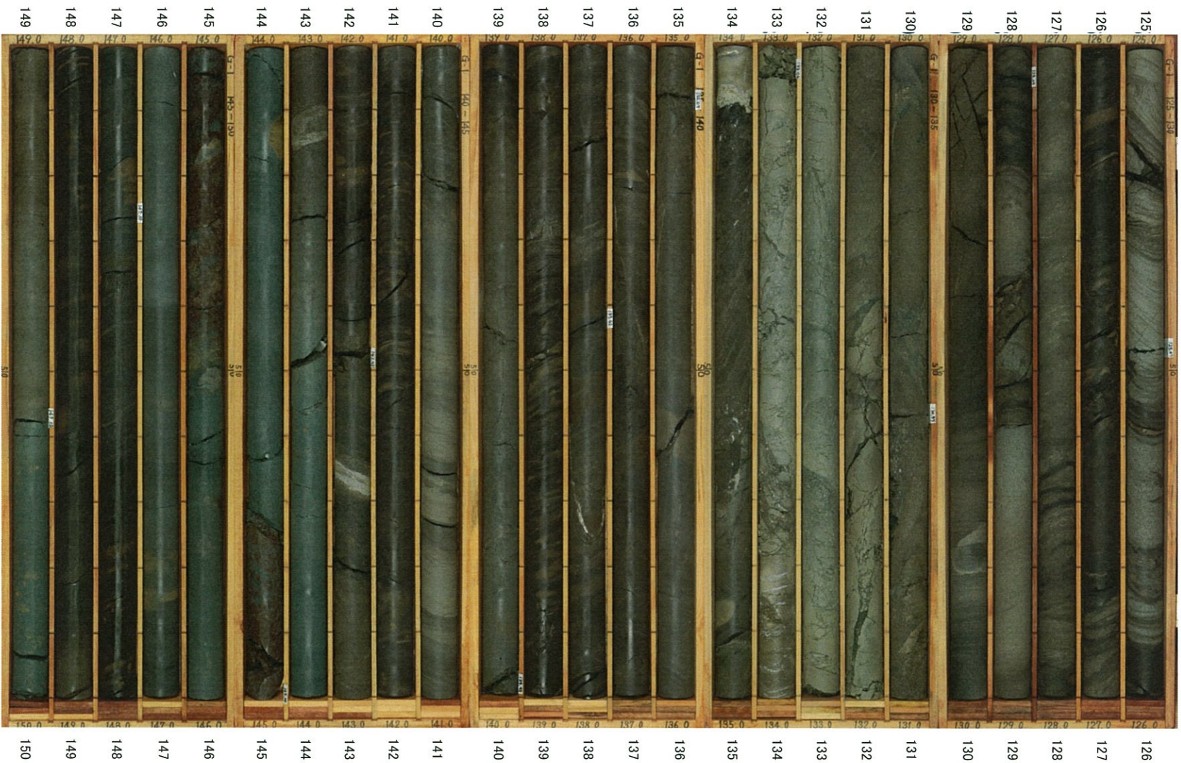
G-1孔 (6/10) 深度125～150m
