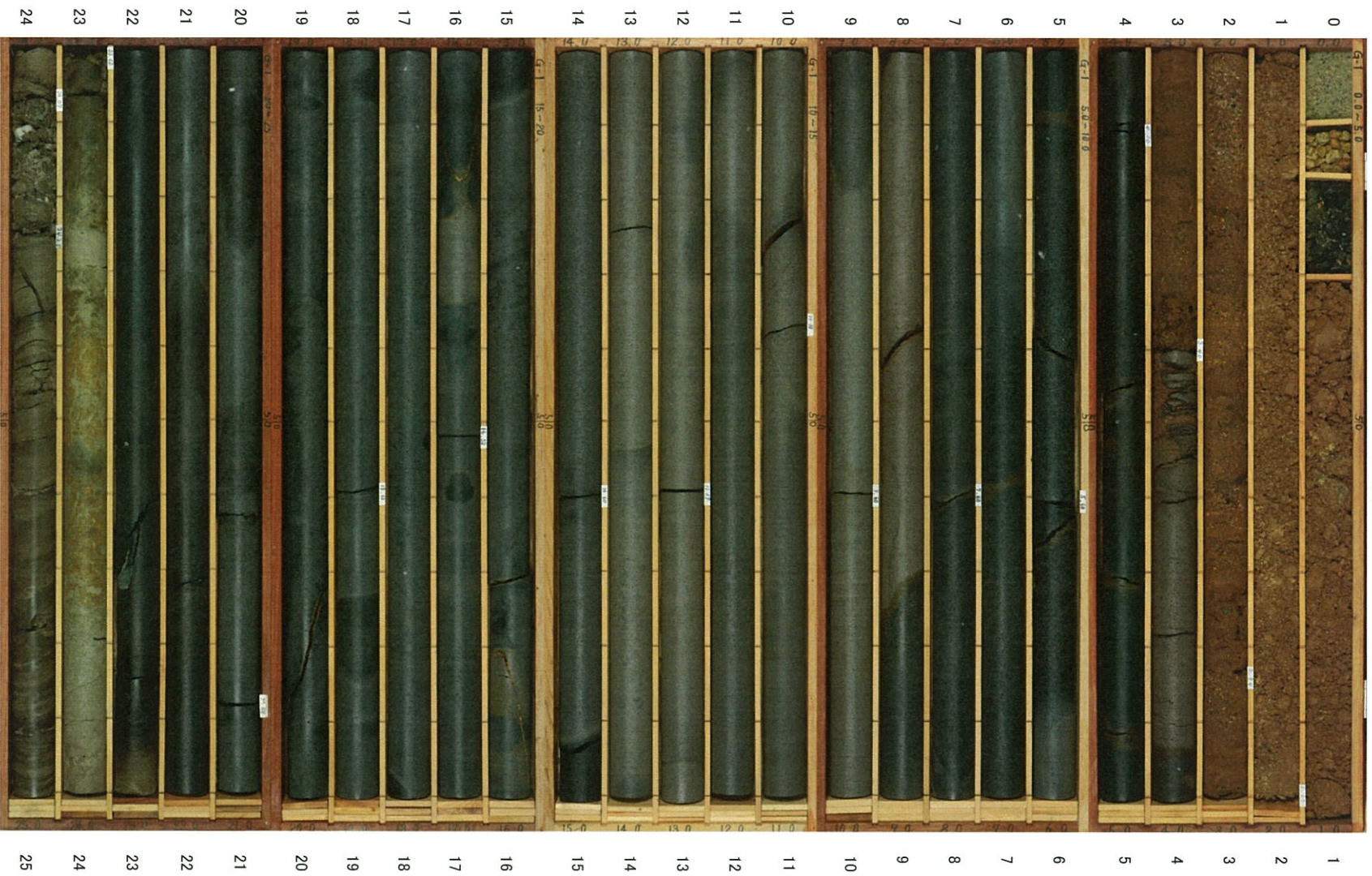
G-1孔 (1/10) 深度0~25m
