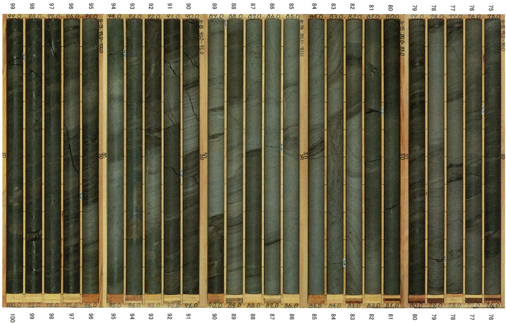
G-15孔(4/8) 深度75~100m
