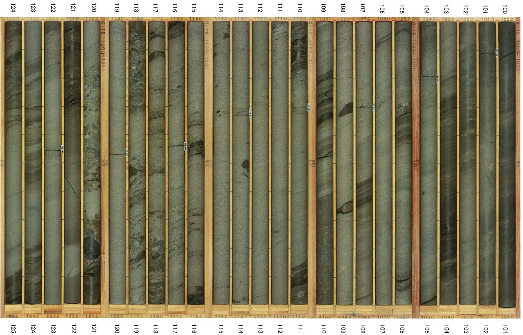
G-12孔 (5/8) 深度100～125m
