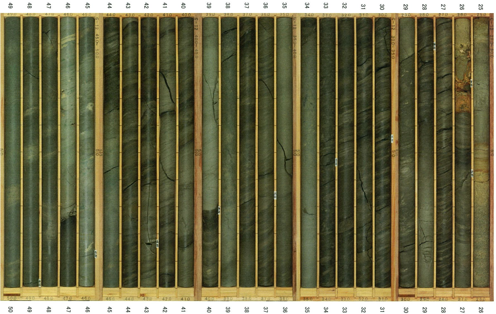
G-12孔(2/8) 深度25～50m
