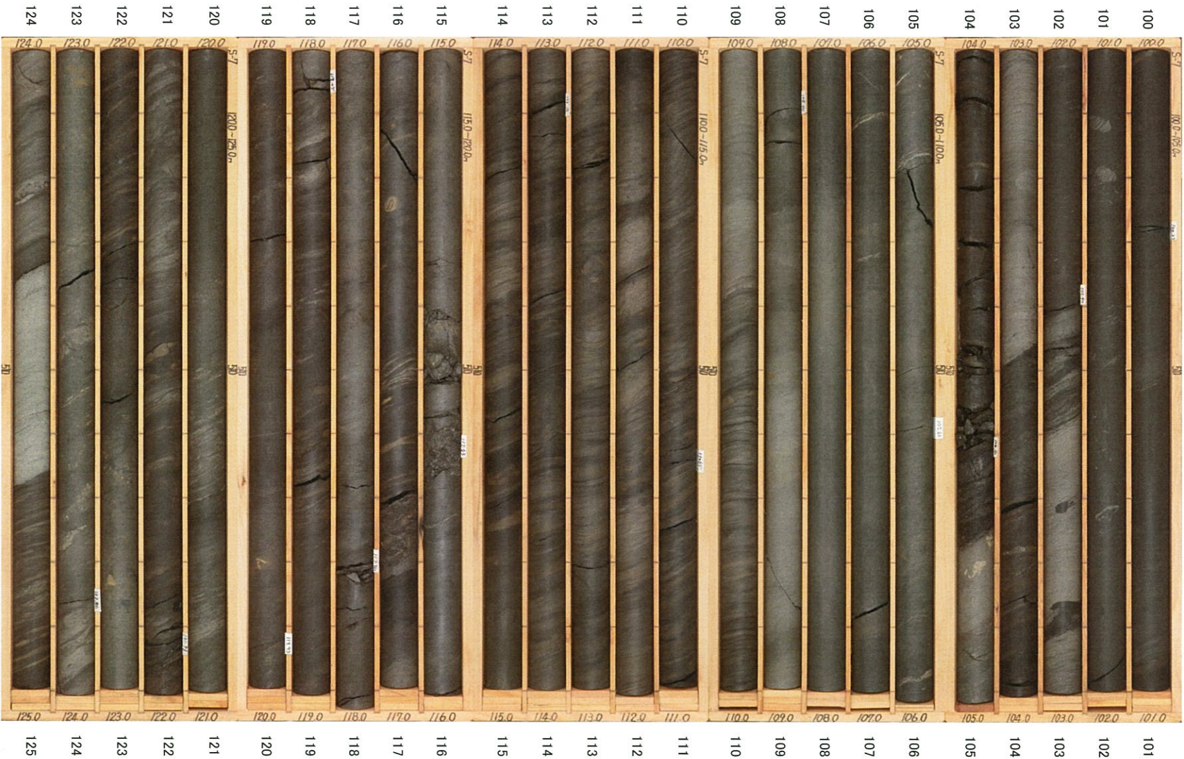
S-7孔 (5/8) 深度100～125m
