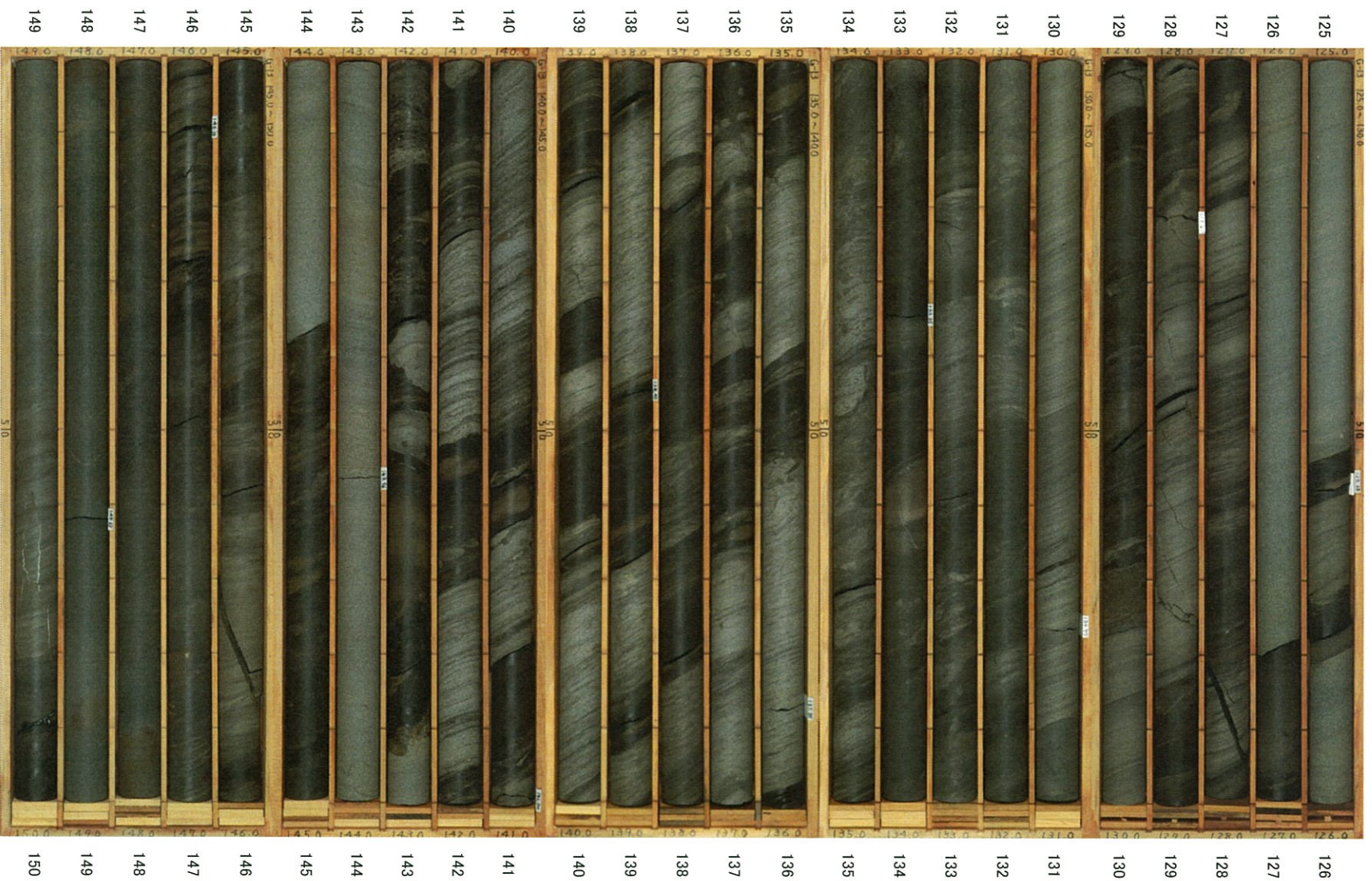
G-13孔(6/8) 深度125～150m
