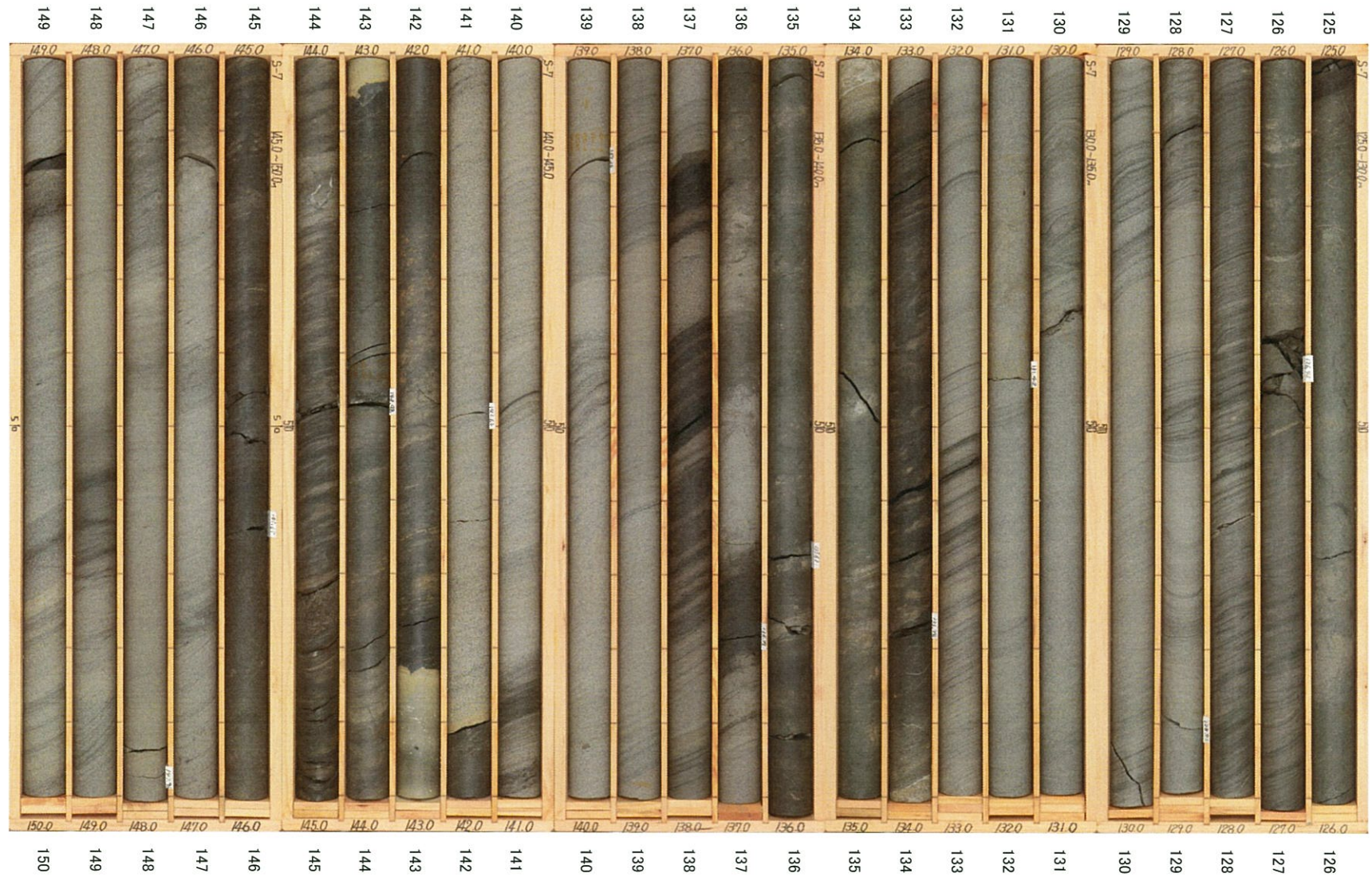
S-7孔(6/8) 深度125~150m
