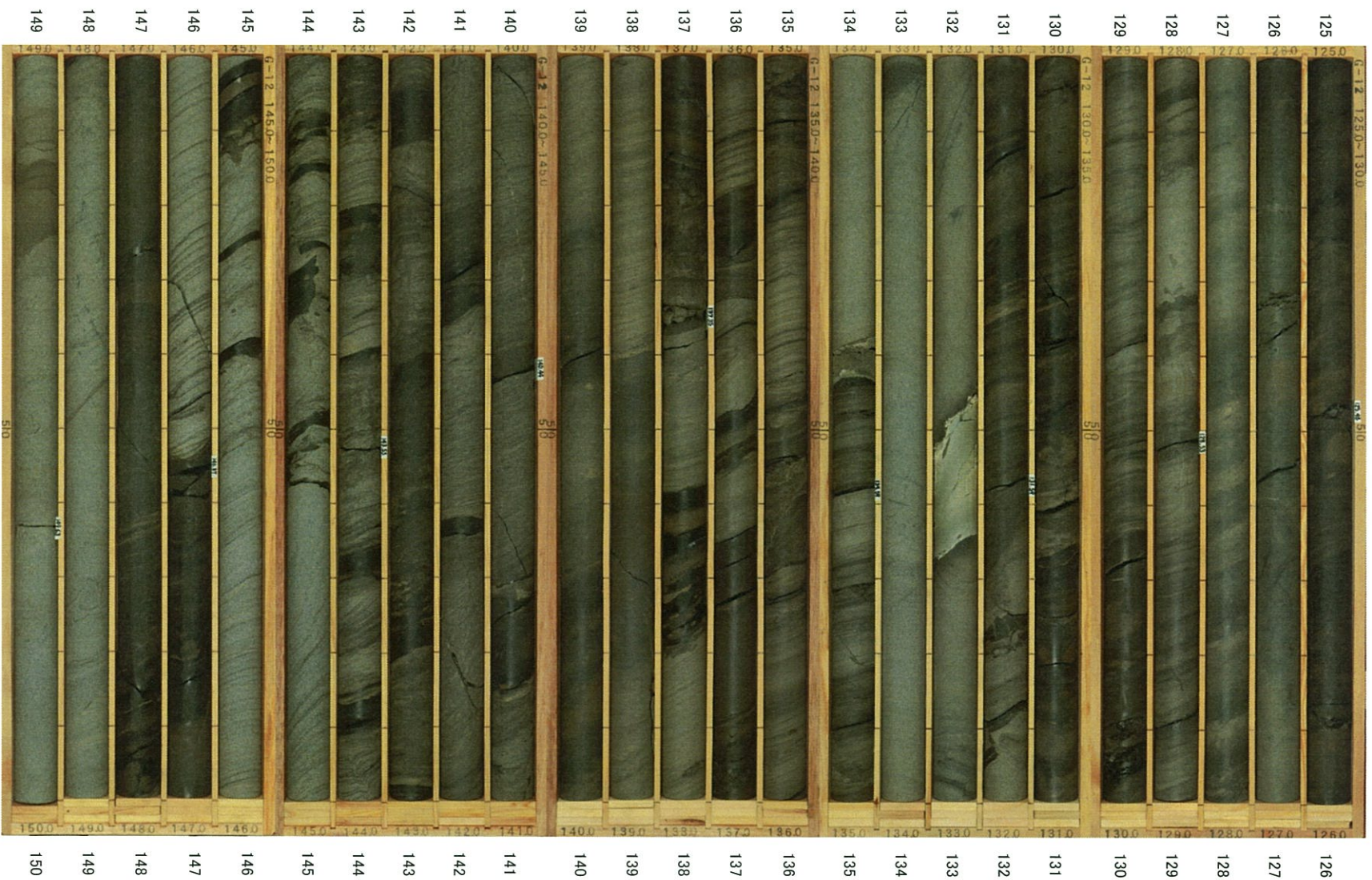
G-12孔 (6/8) 深度125～150m
