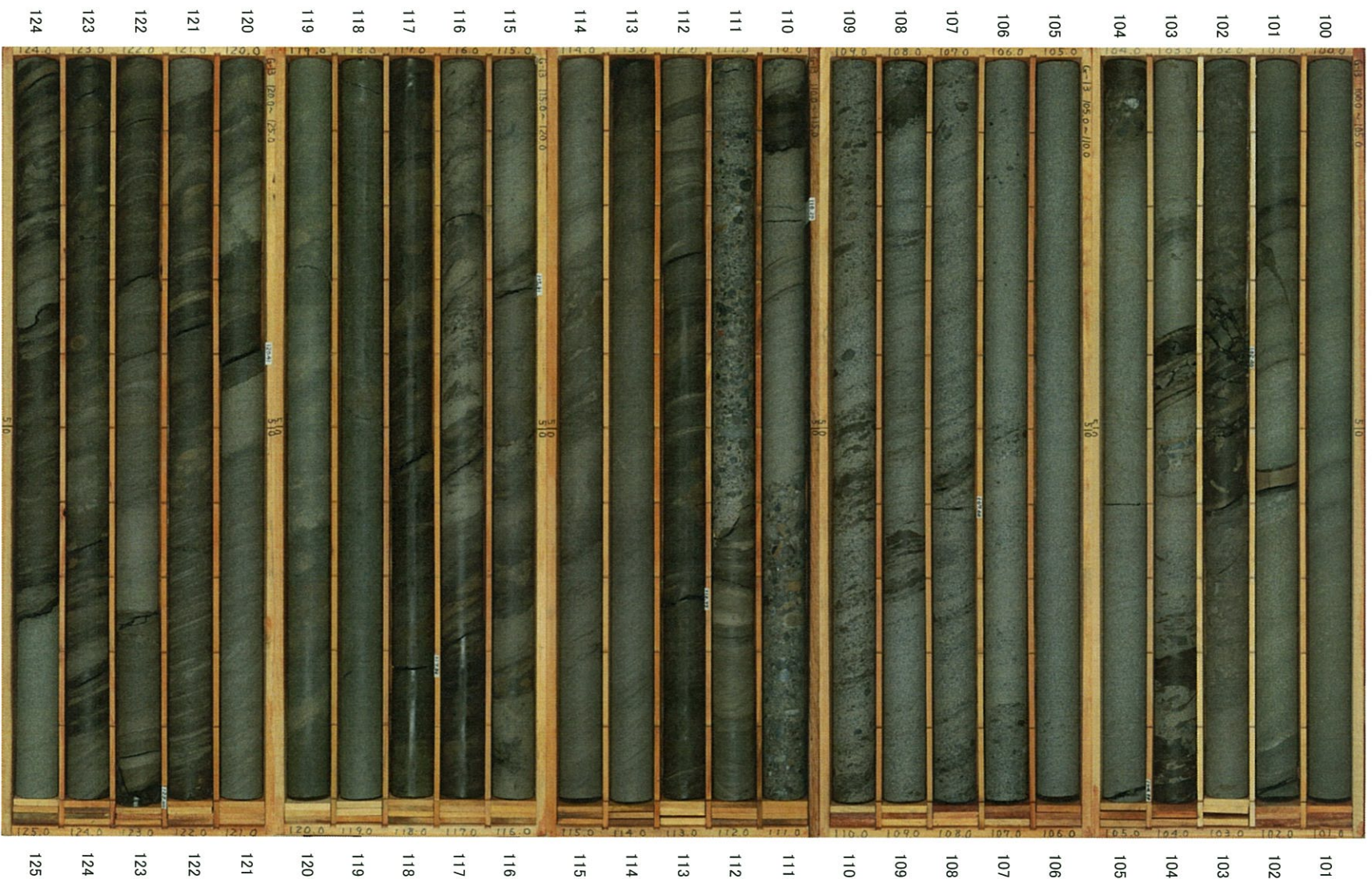
G-13孔 (5/8) 深度100～125m
