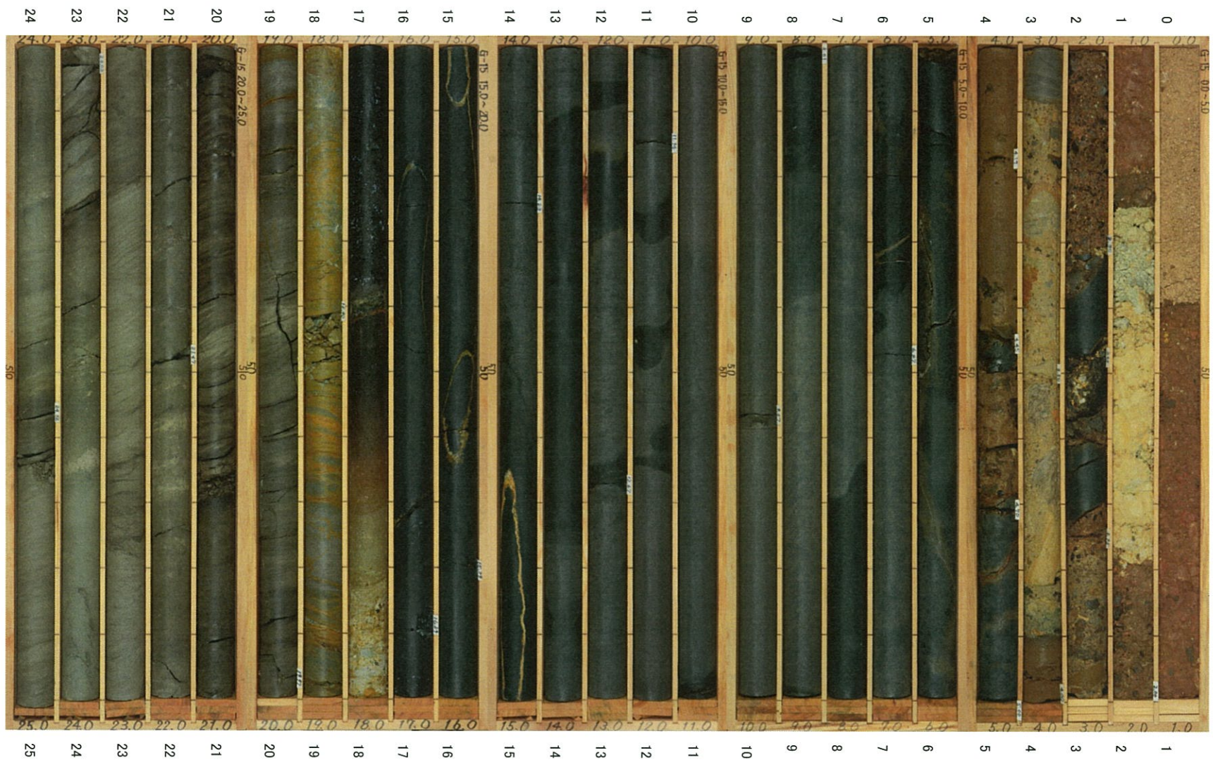
G-15孔 (1/8) 深度0~25m
