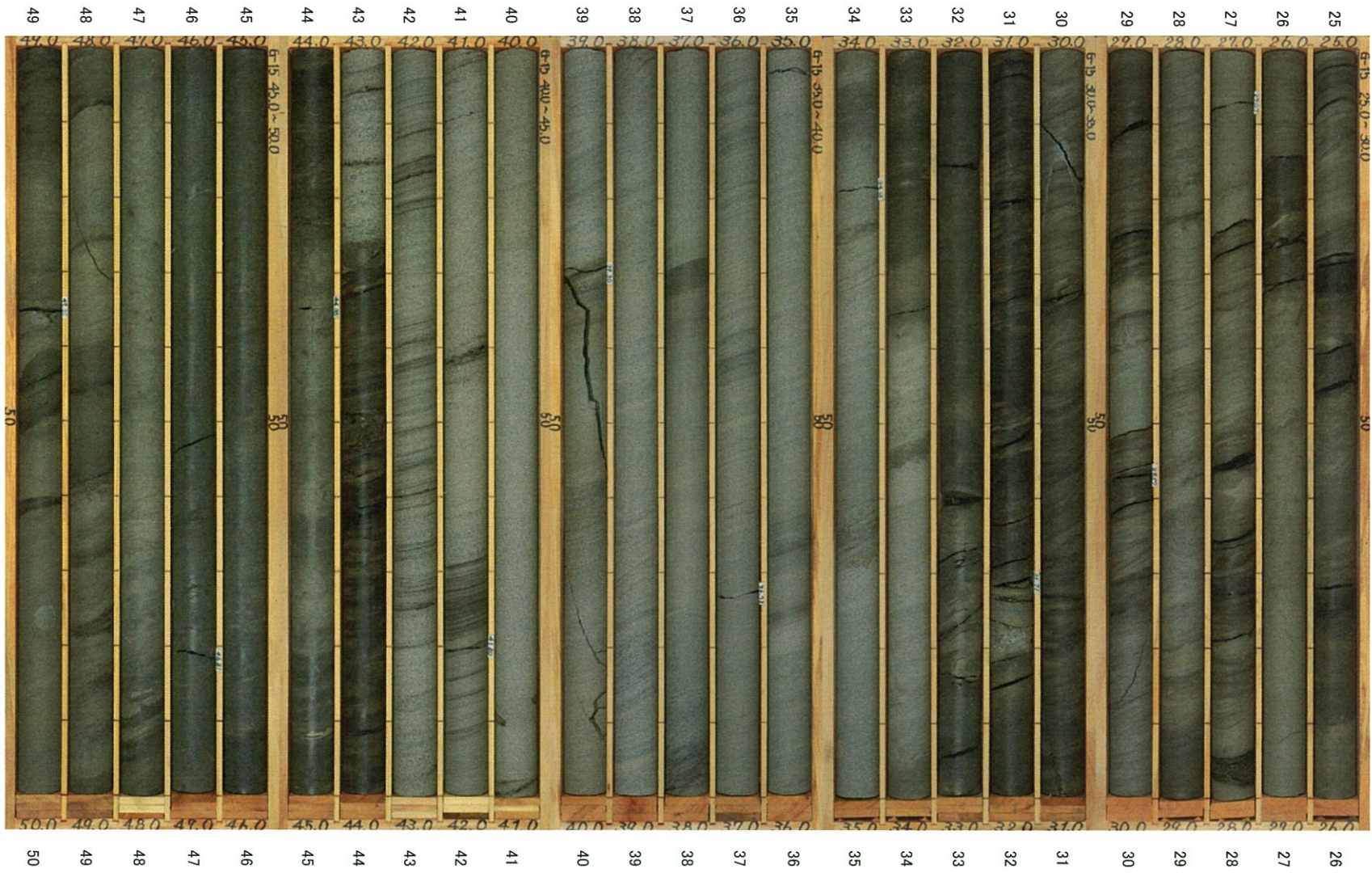
G-15孔(2/8) 深度25~50m
