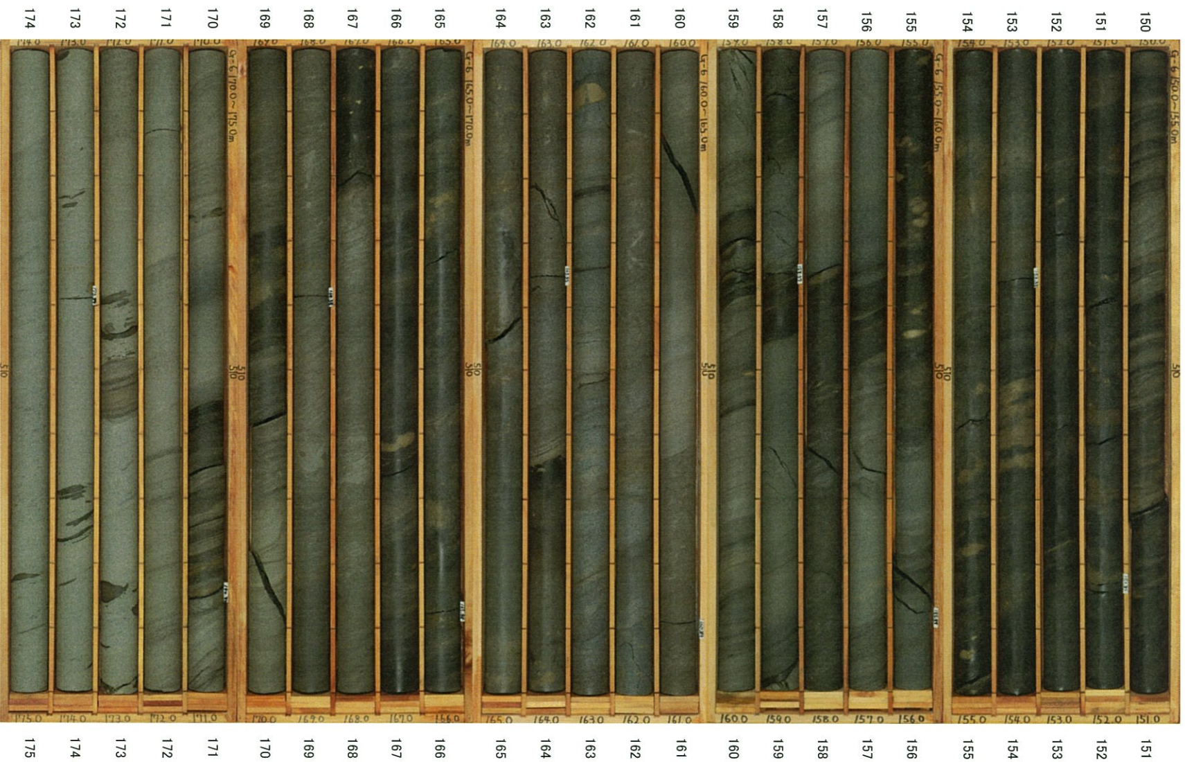
G-6孔 (7/8) 深度150～175m
