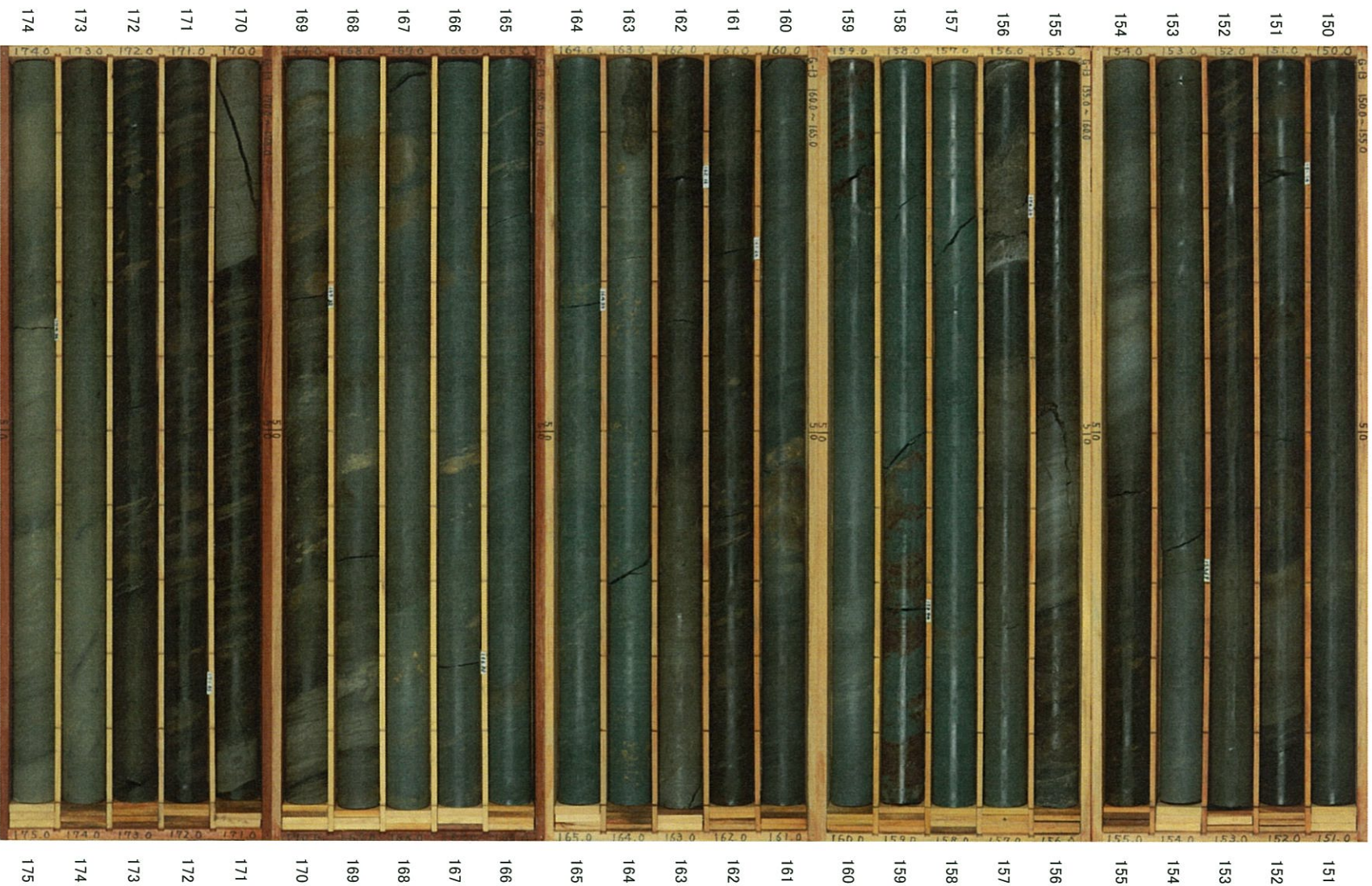
G-13孔 (7/8) 深度150~175m
