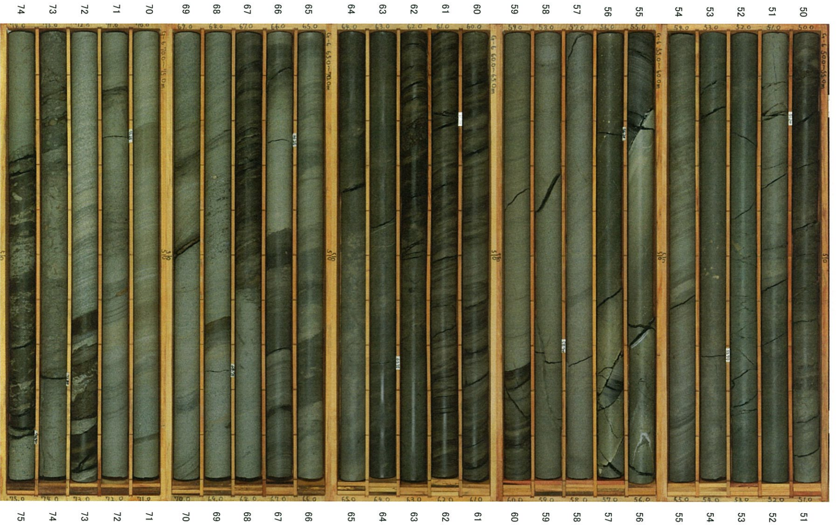
G-6孔 (3/8) 深度50～75m
