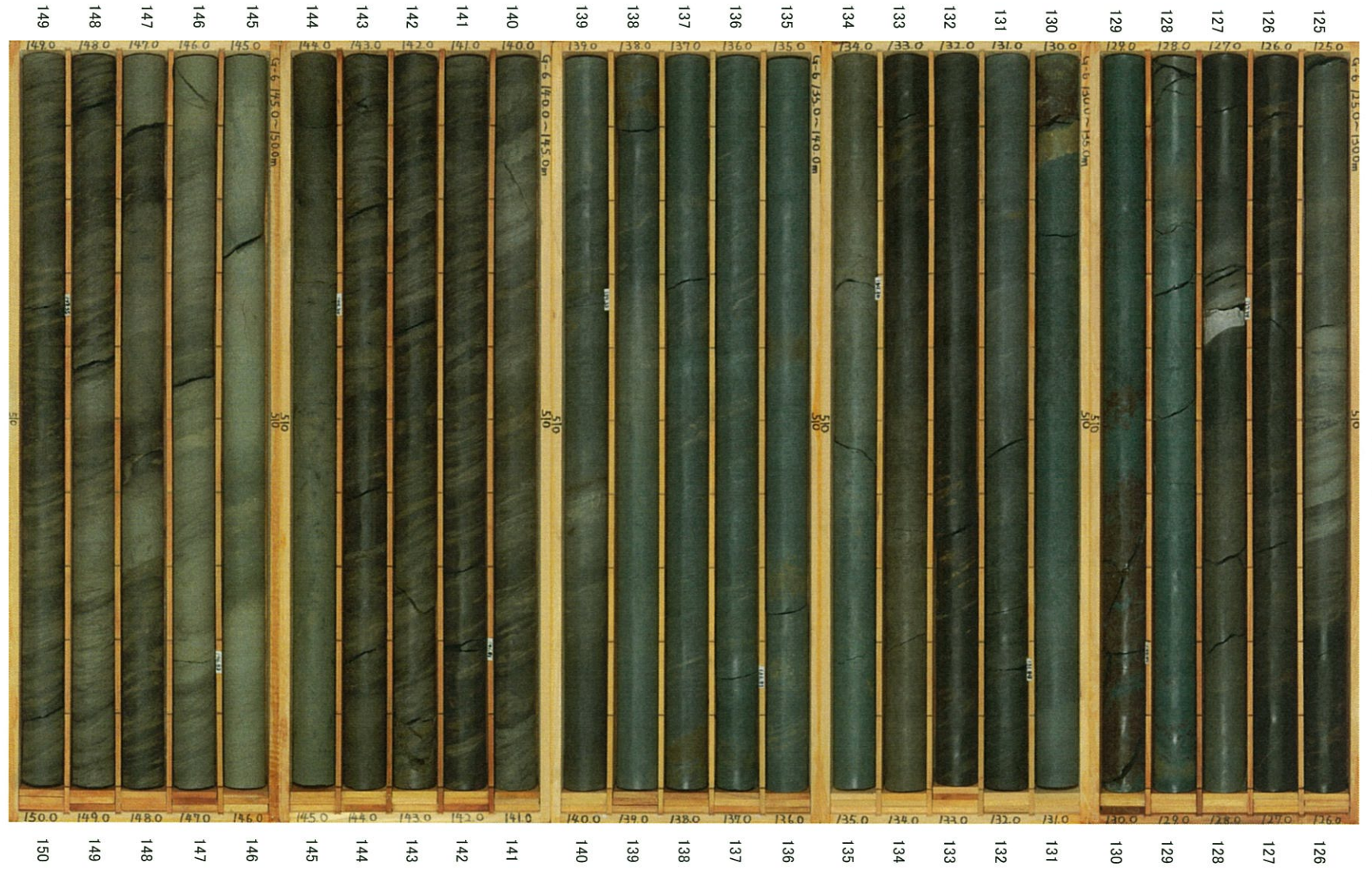
G-6孔 (6/8) 深度125～150m
