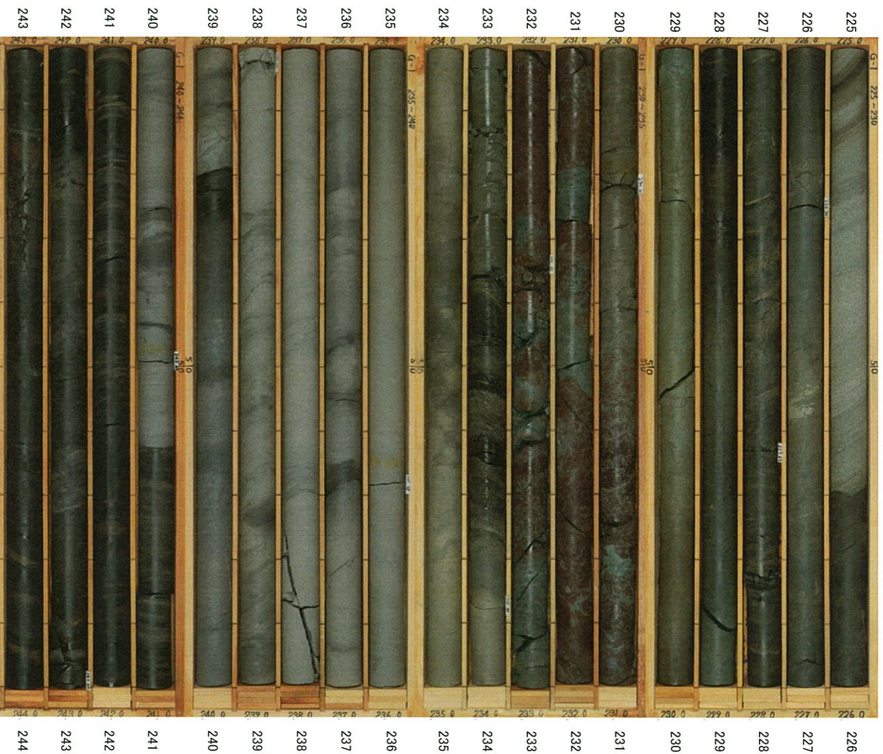
G-1孔 (10/10) 深度225～244m
