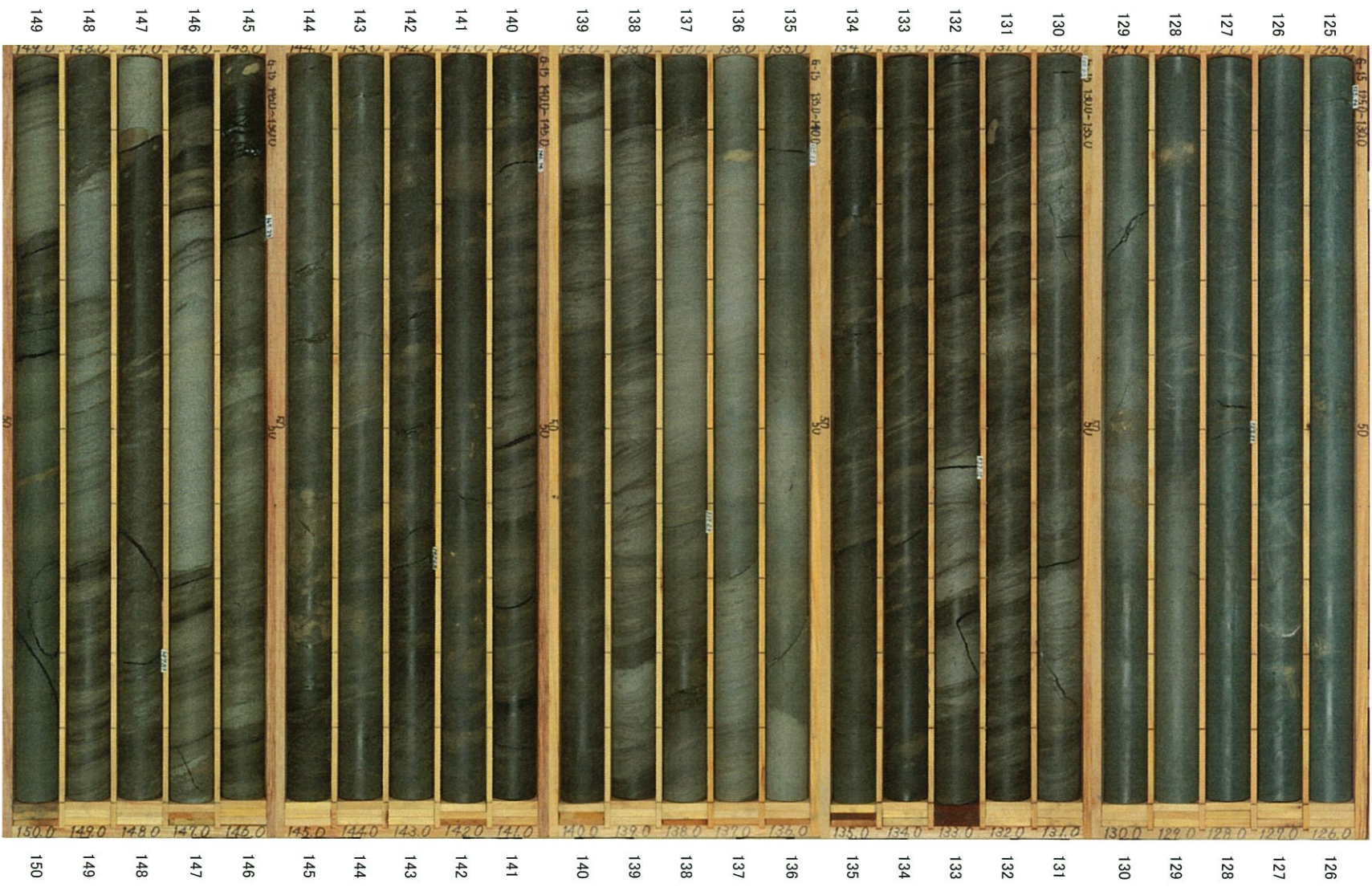
G-15孔(6/8) 深度125～150m
