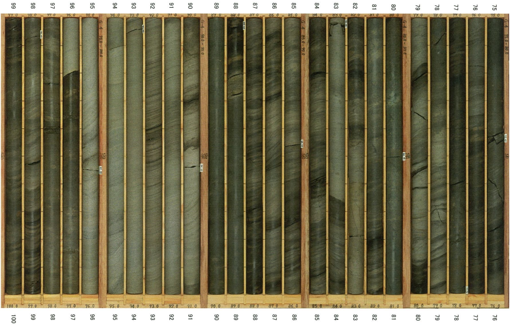
G-4孔 (4/8) 深度75~100m
