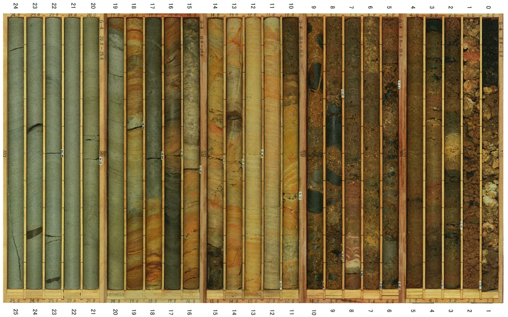
G-4孔 (1/8) 深度0~25m
