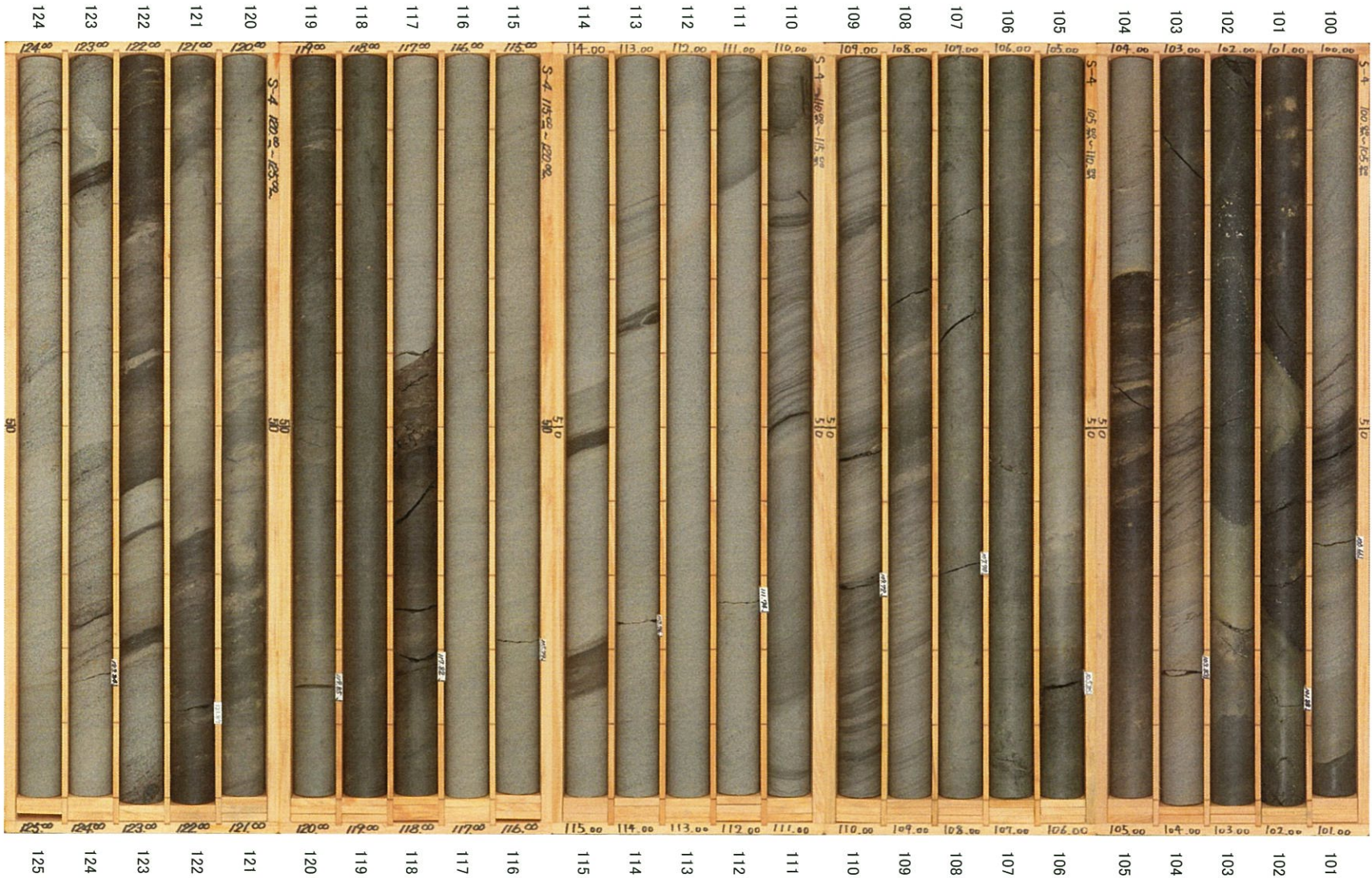
S-4孔 (5/6) 深度100～125m
