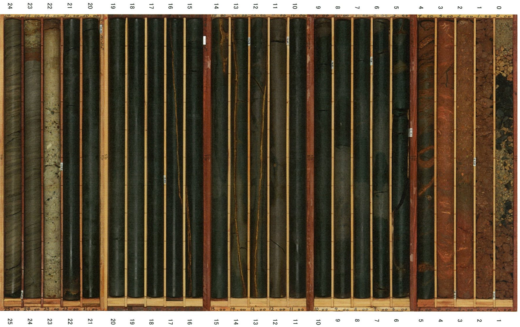
G-14孔(1/8) 深度0~25m
