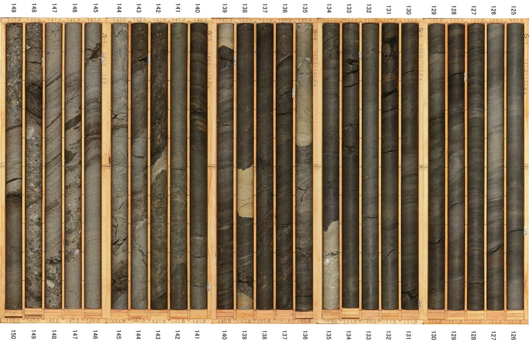
S-5孔(6/8) 深度125～150m
