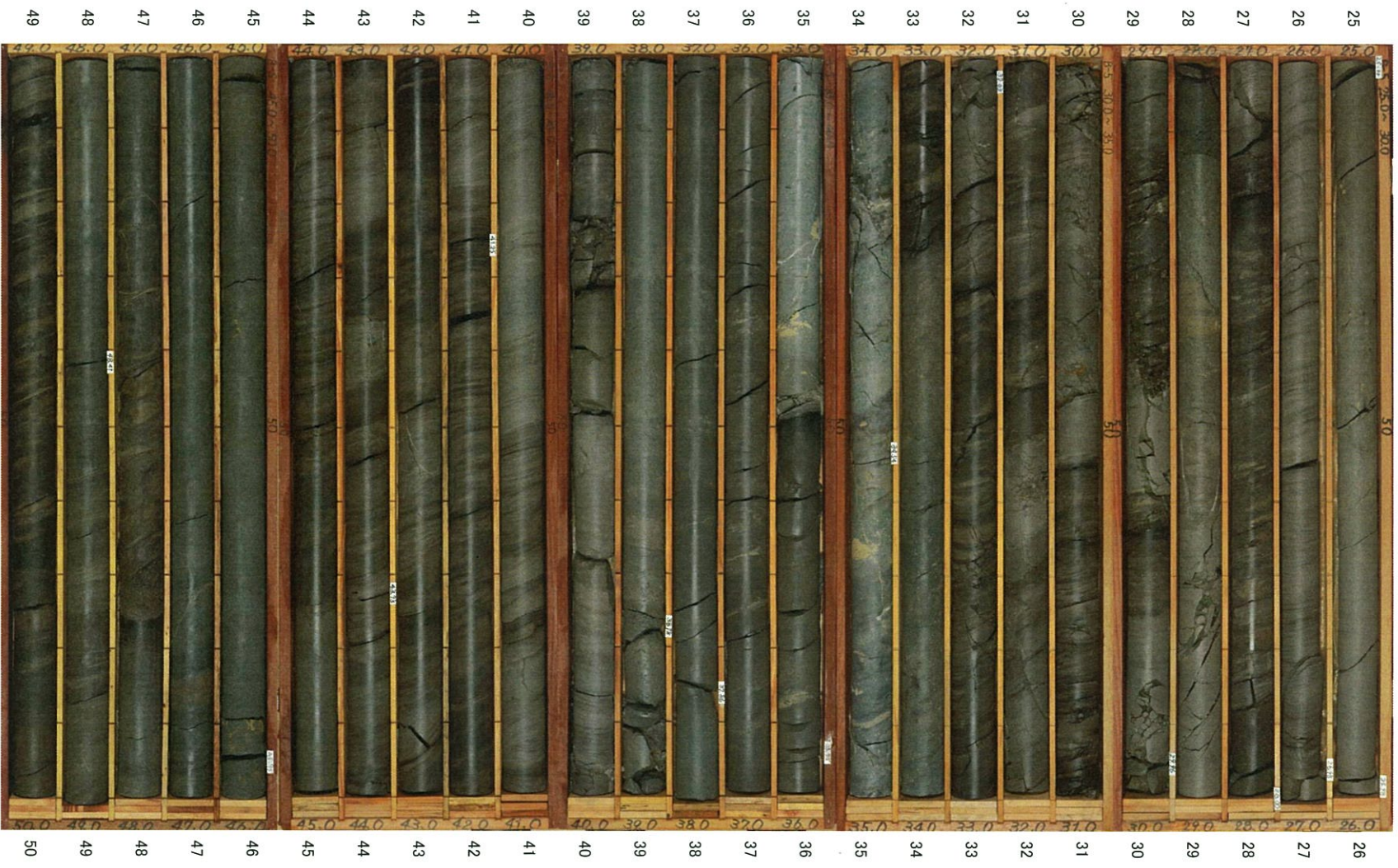
B-5孔 (2/6) 深度25～50m
