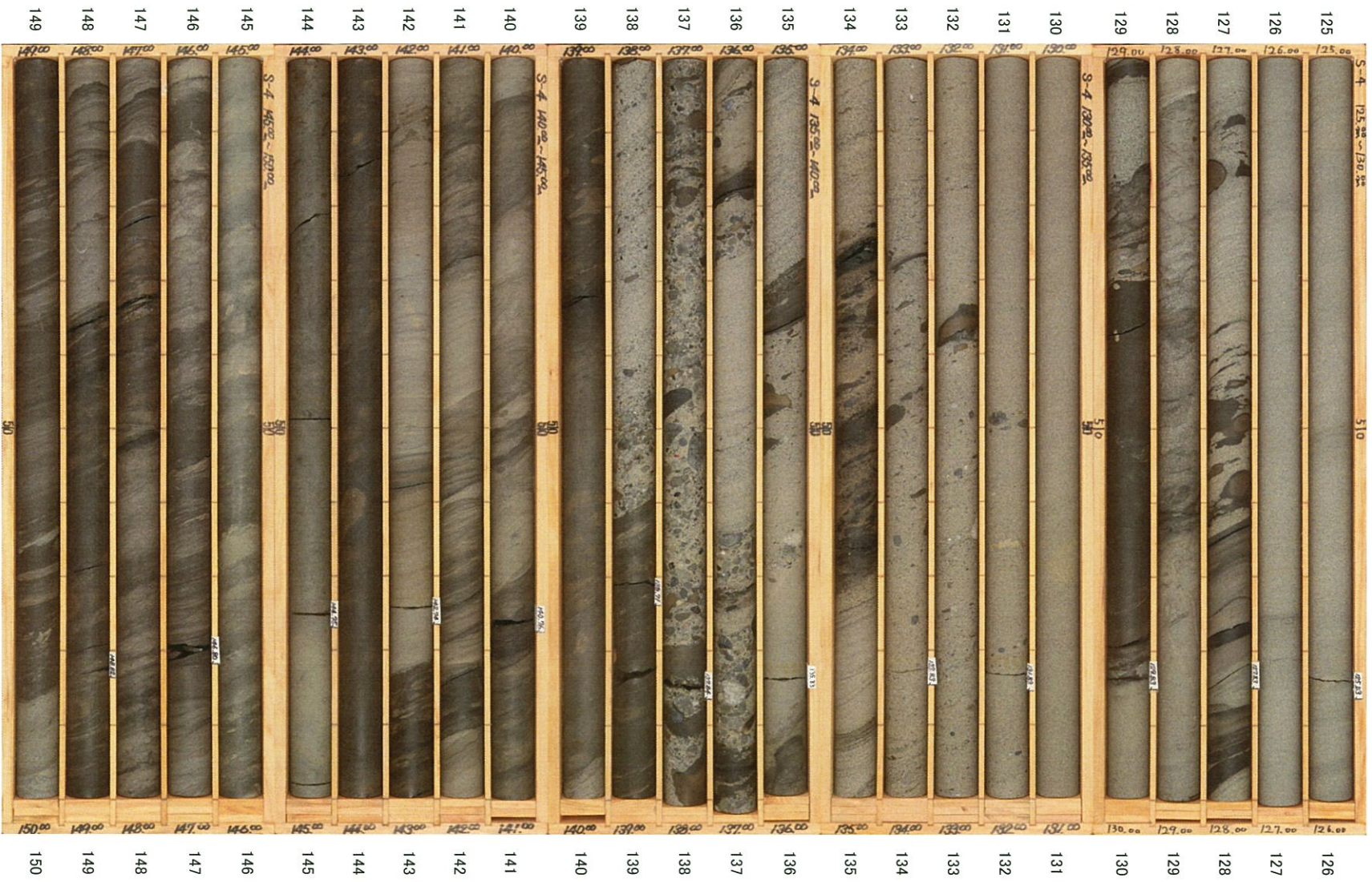
S-4孔 (6/6) 深度125～150m
