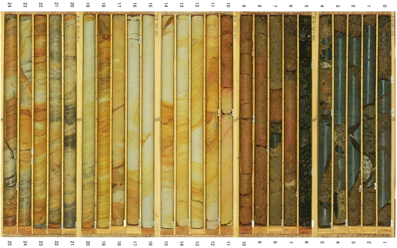
B-15孔 (1/3) 深度0~25m
