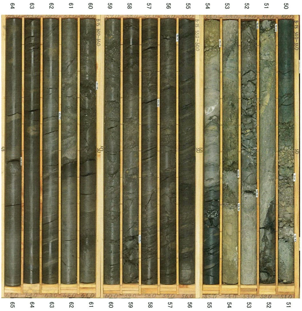
B-15孔 (3/3) 深度50～65m
