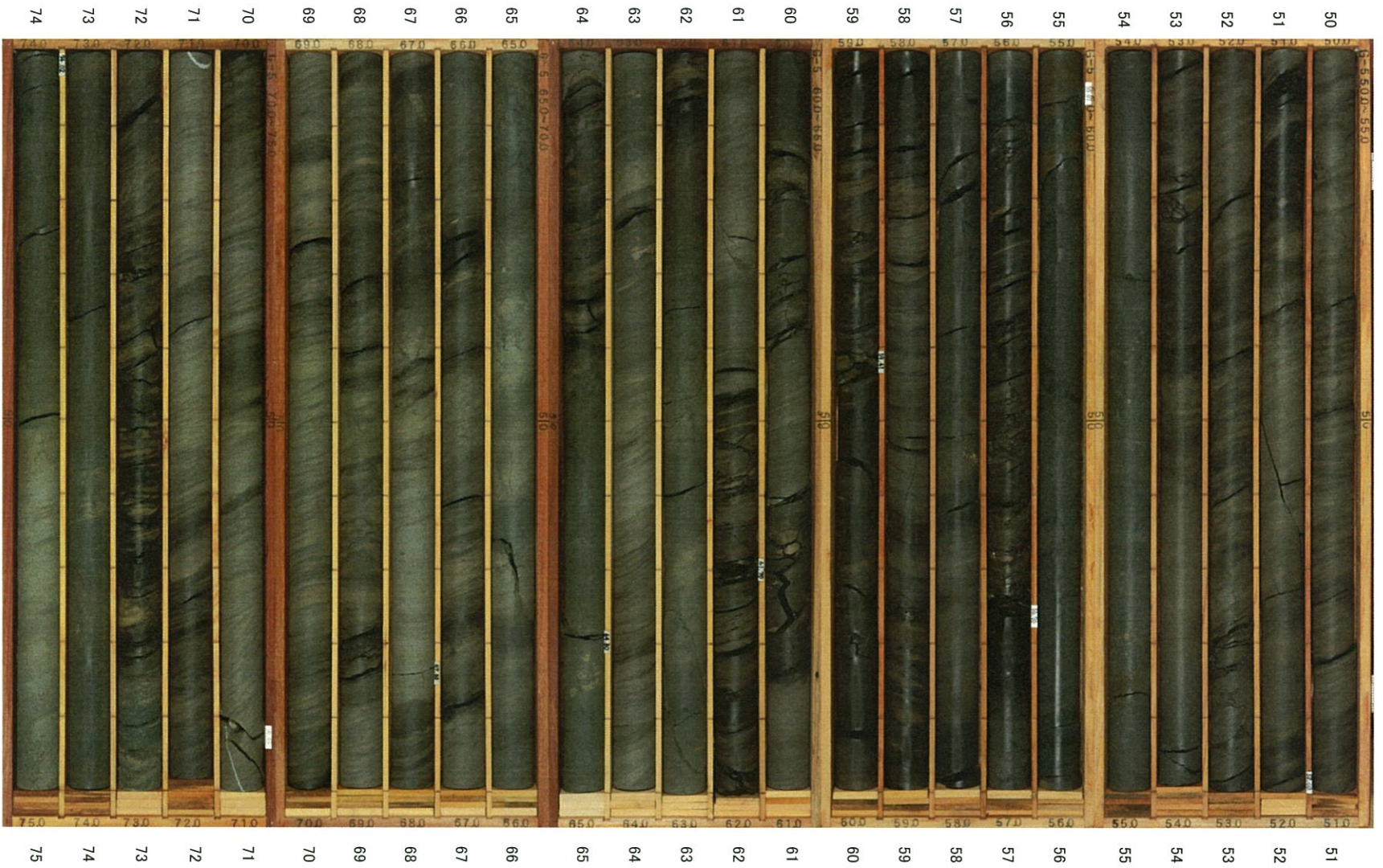
G-5孔 (3/8) 深度50～75m
