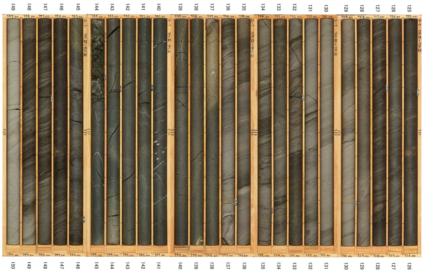
S-1孔 (6/6) 深度125～150m
