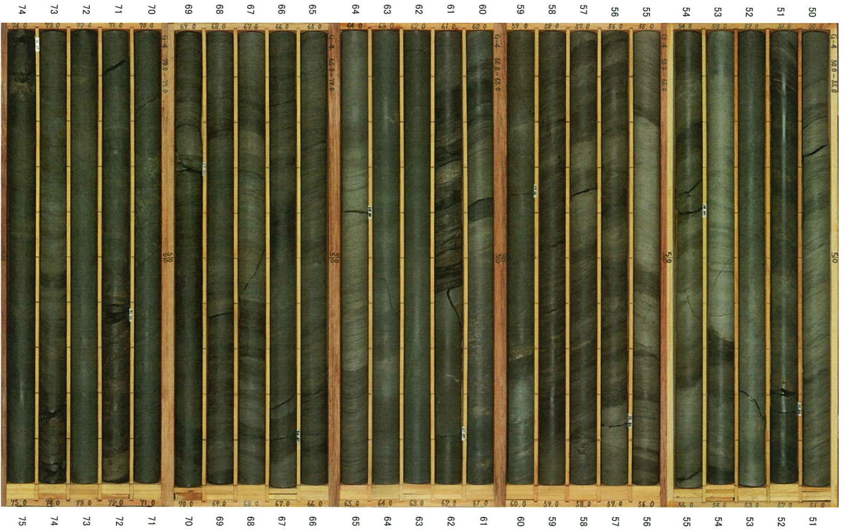
G-4孔 (3/8) 深度50～75m
