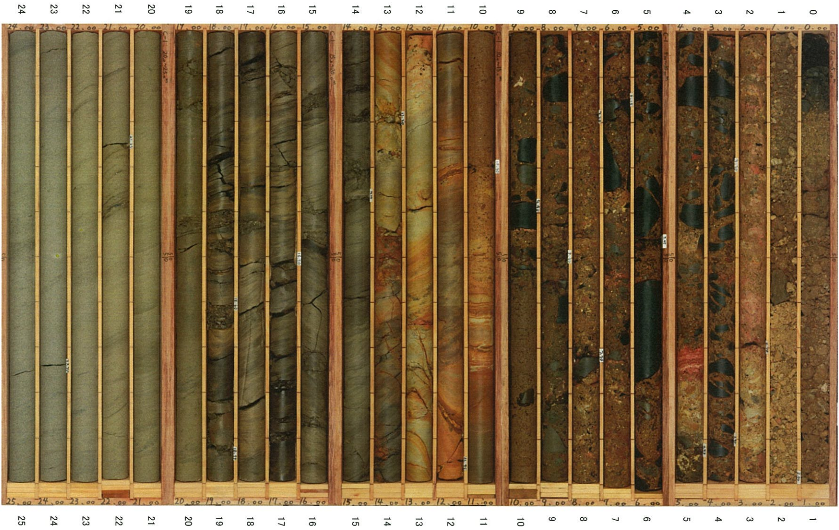
C-1孔(1/6) 深度0~25m
