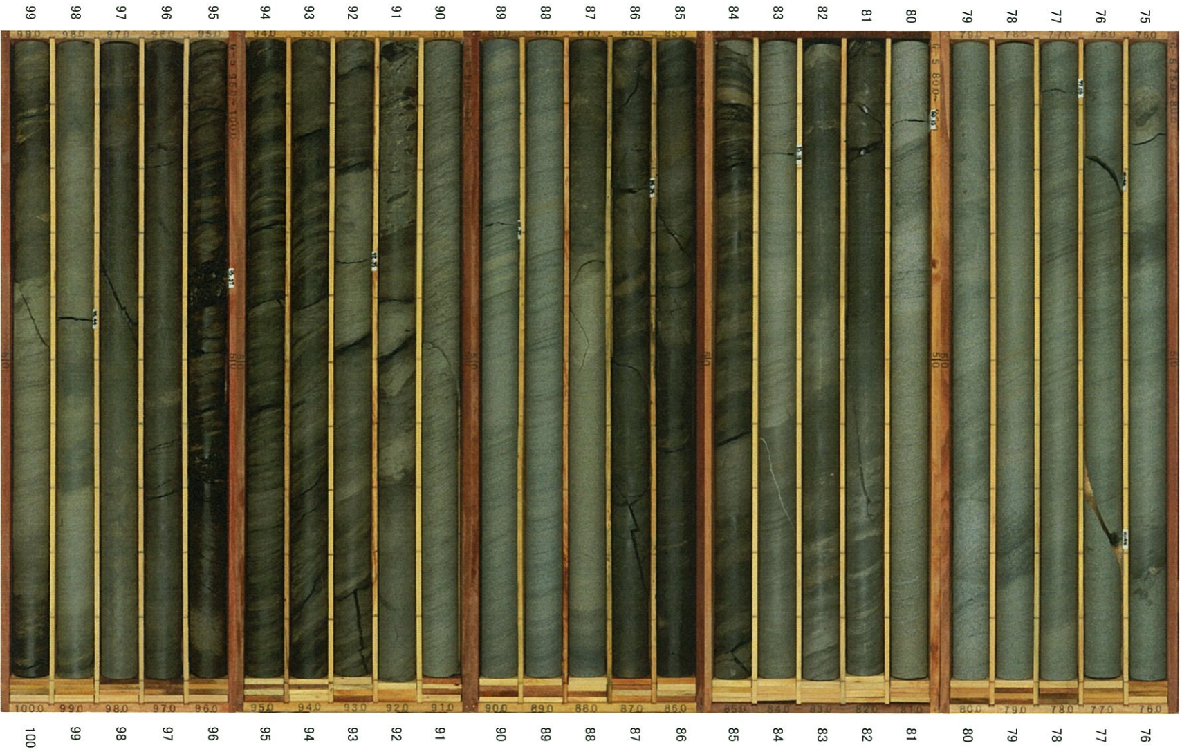
G-5孔 (4/8) 深度75~100m
