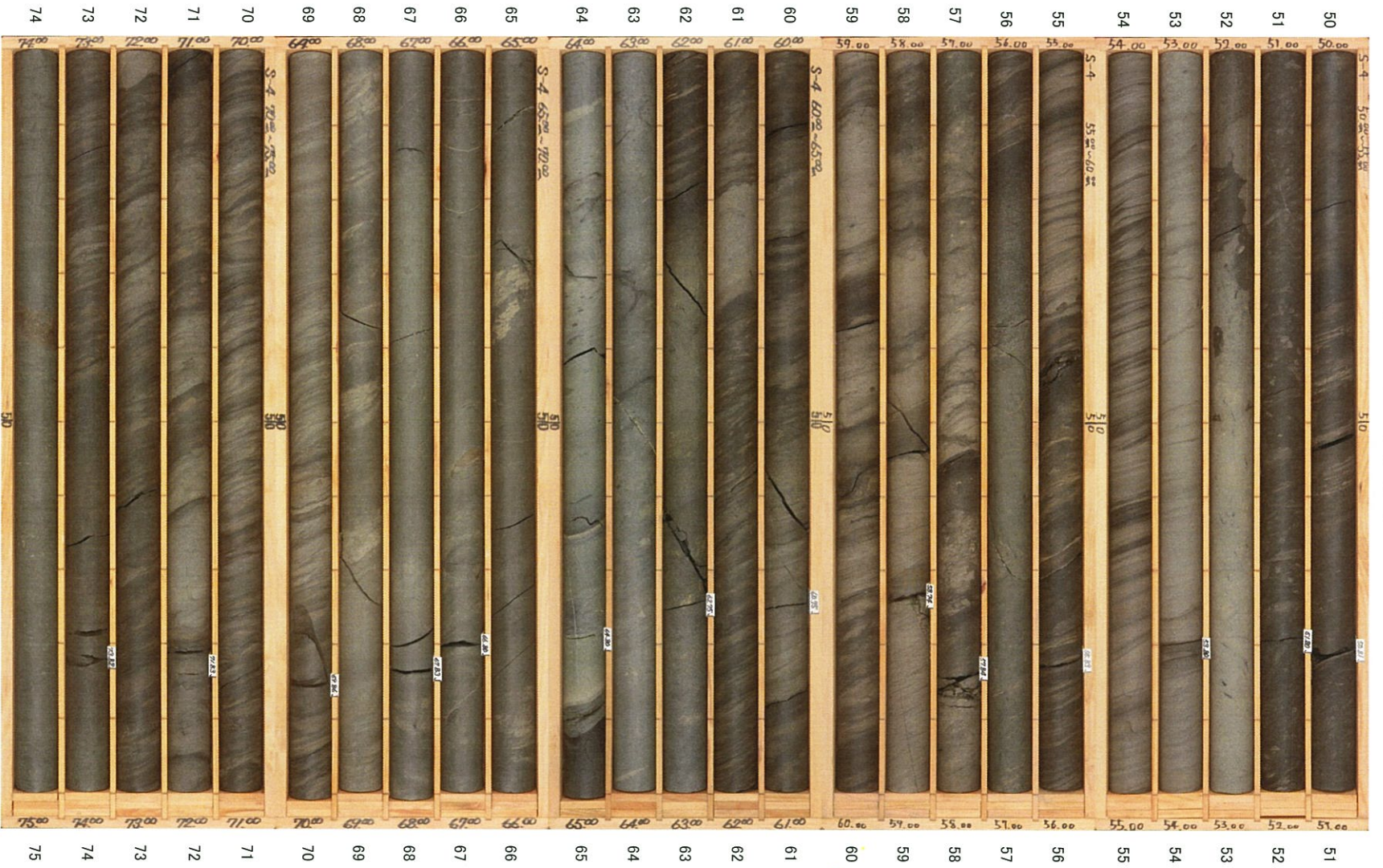
S-4孔 (3/6) 深度50～75m
