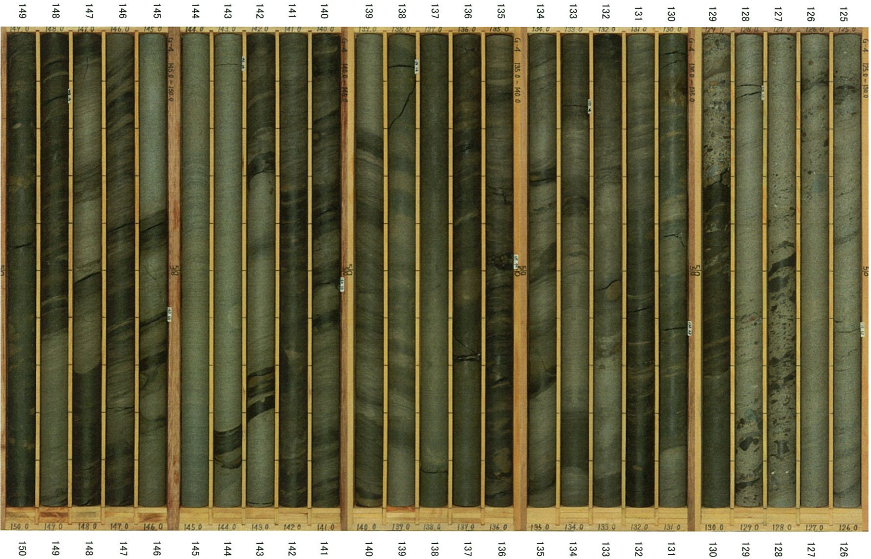
G-4孔 (6/8) 深度125～150m
