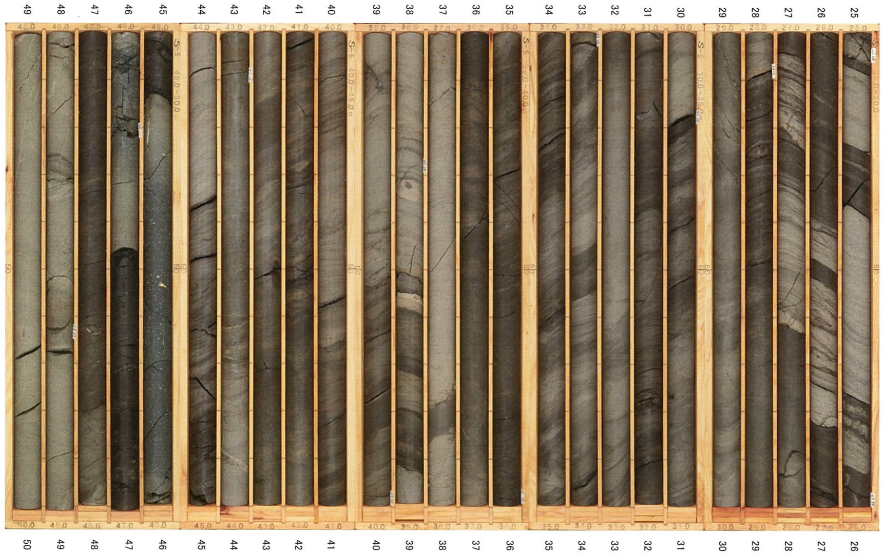
S-5孔 (2/8) 深度25～50m
