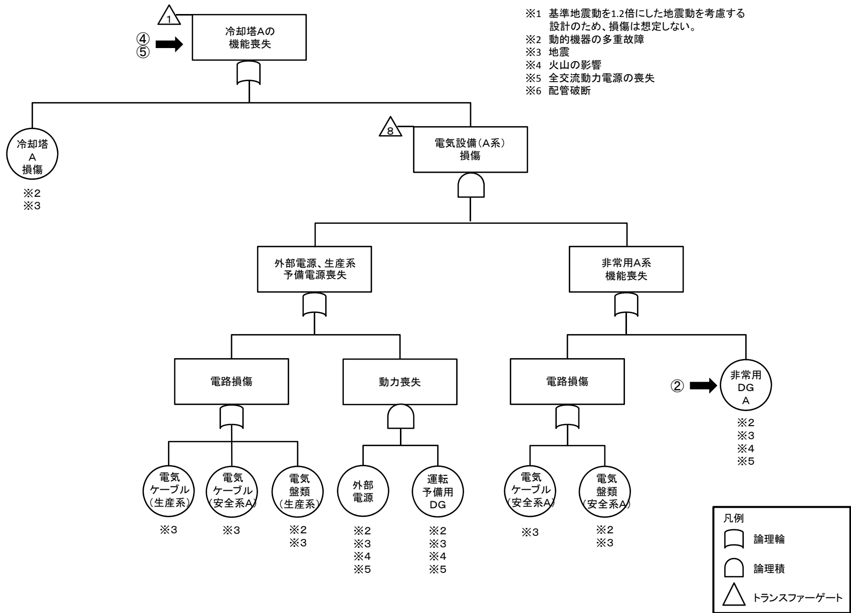
第1.2-1図 蒸発乾固の発生の防止のための措置の機能喪失原因対策分析(11/15)
