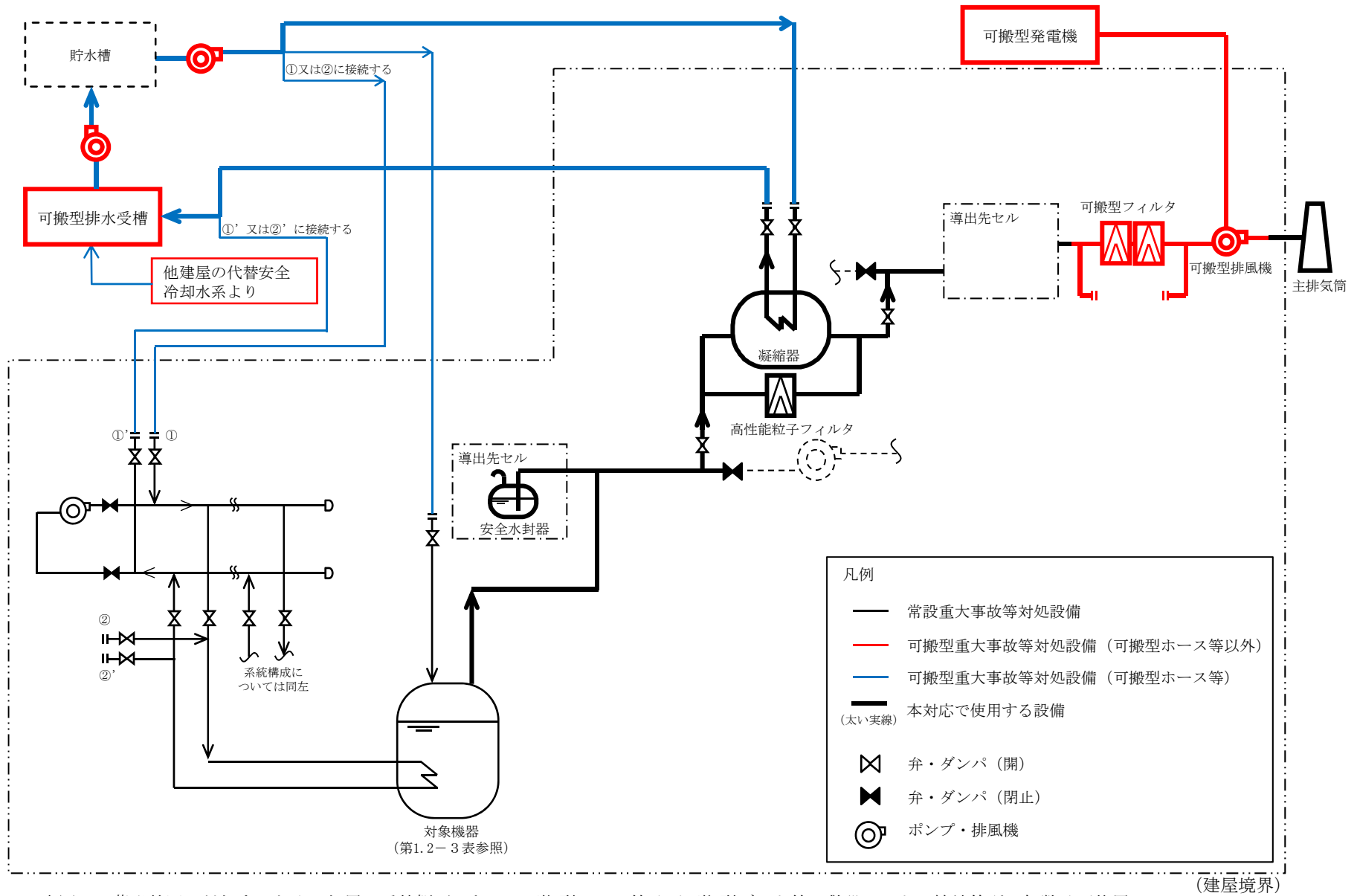
第1.2-32図 セルへの導出経路の構築及びセル排気系を代替する排気系による対応の系統概要図
