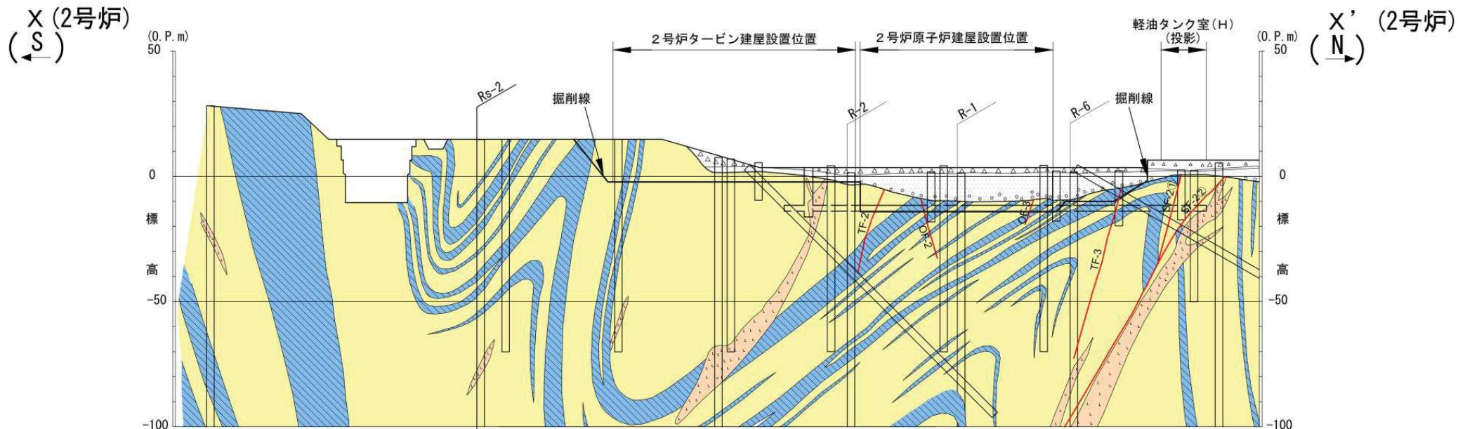
2号炉X-X'断面(交差断面)
