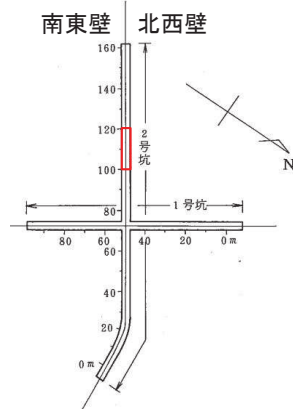
試掘坑配置図
