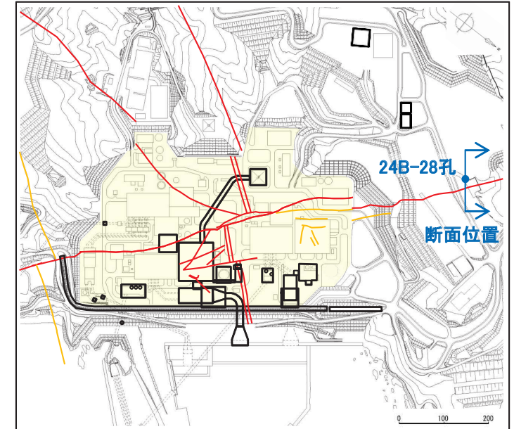
ボーリング位置図(24B-28孔)
