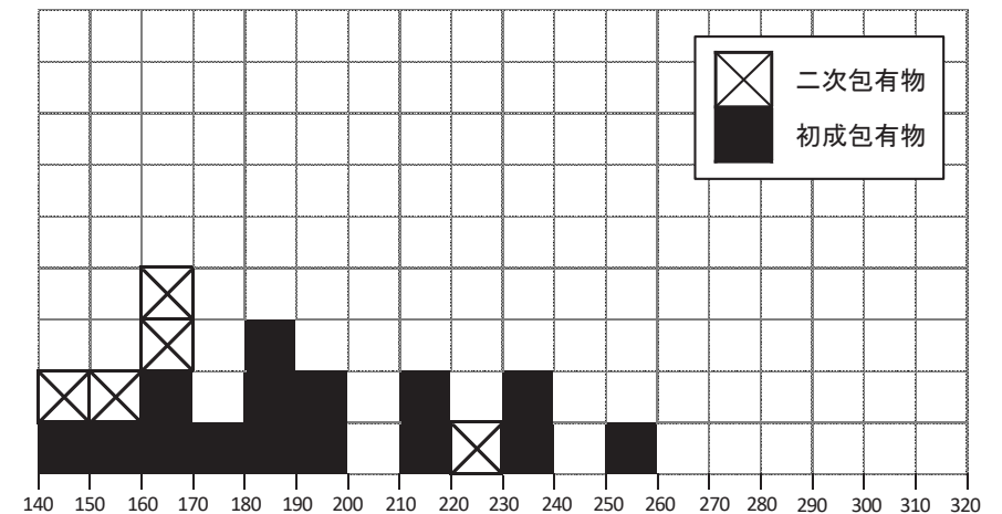
均質化温度の分布図(ヒストグラム)
