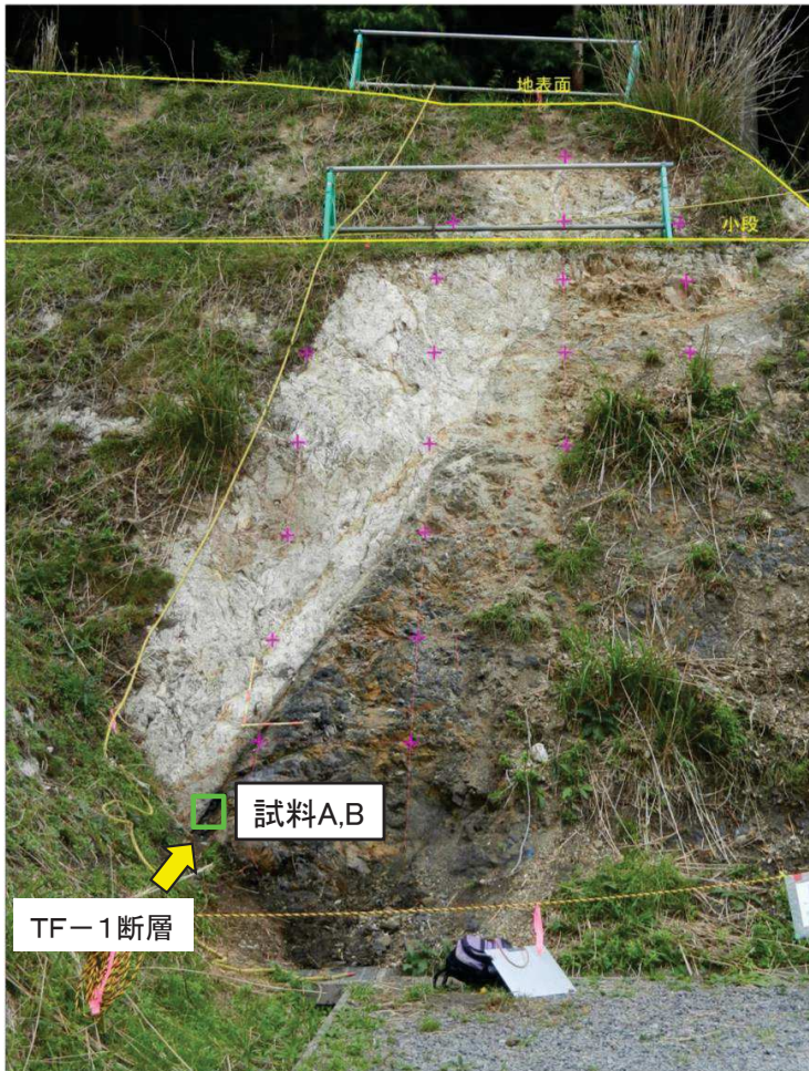
TF-1断層露頭写真
