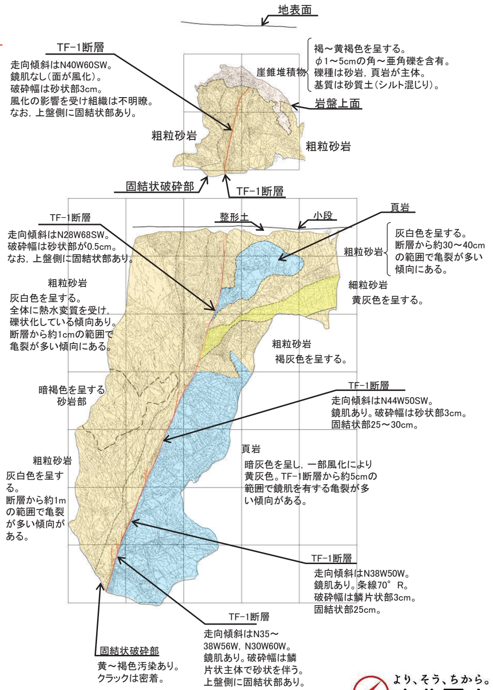
TF-1断層露頭スケッチ
