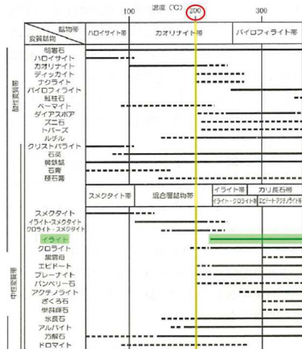
※日本粘土学会編(2009)
