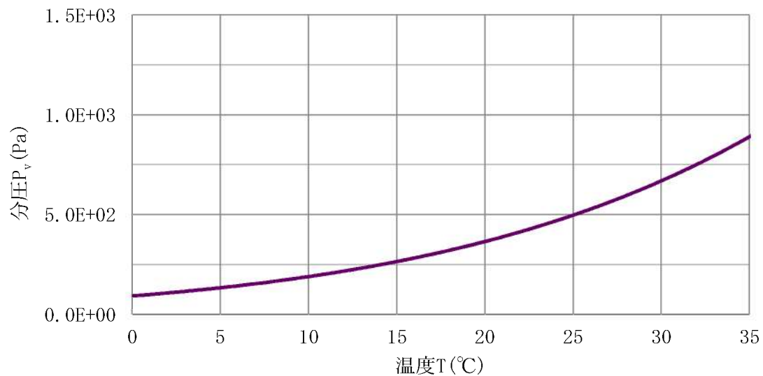
図2 ヒドラジン (38.4wt%) の分圧曲線
